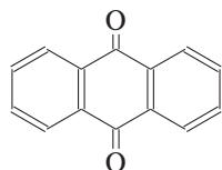
9,10-антрахинон
