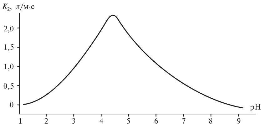
Рис.16.3. Зависимость скорости образования оксима ацетона от рН
