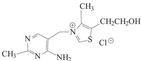
тиаминхлорид (витамин B 1 )
