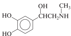
адреналин
