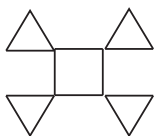
4-ротан
