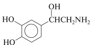
норадреналин
