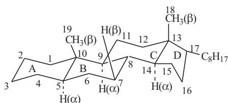
5 \alpha -холестан
