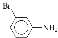
3-бромбензоламин
