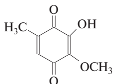
3-гидрокси-2-метокси- 5-метил-1,4-бензохинон (антибиотик фумигатин)
