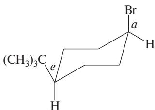
цис -4-бром-1- трет -бутил циклогексан
