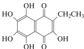
эхинохром А (пигмент морского ежа)
