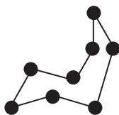
ванна-кресло
