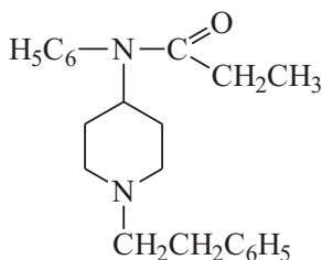
фентанил
