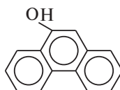
9-фенантрол
