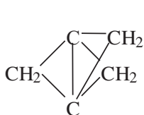
[1,1,1]-пропеллан
