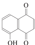
юглон (5-гидро- кси-1,4-нафтохинон)
