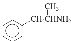
фенамин (амфетамин)
