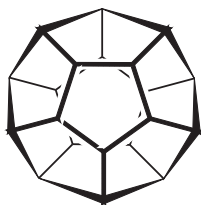
додекаэдран, т. пл. 430°C
