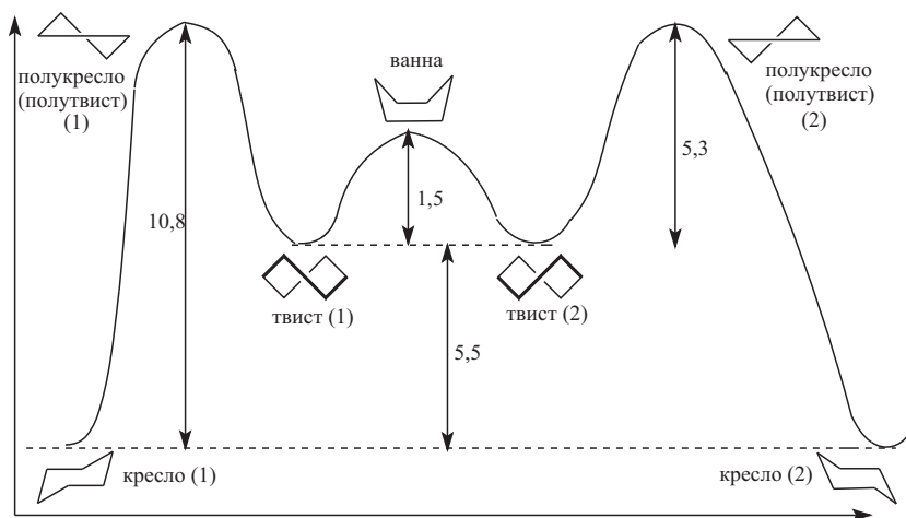
Рис. 22.2. Энергетическая диаграмма конформационных переходов в циклогексане
