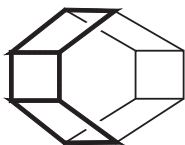
тетрастиран
