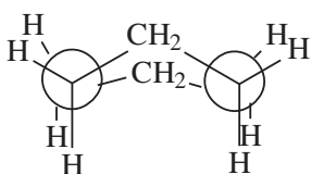
проекция Ньюмена для формы ванны
