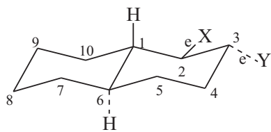
экваториальный ( 2\beta ; 3\alpha )*
