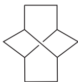
твистан
