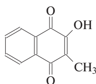
фтиокол (антибиотик) 2-гидрокси-3-метил- 1,4-нафтохинон
