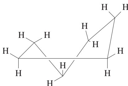
твист-форма
