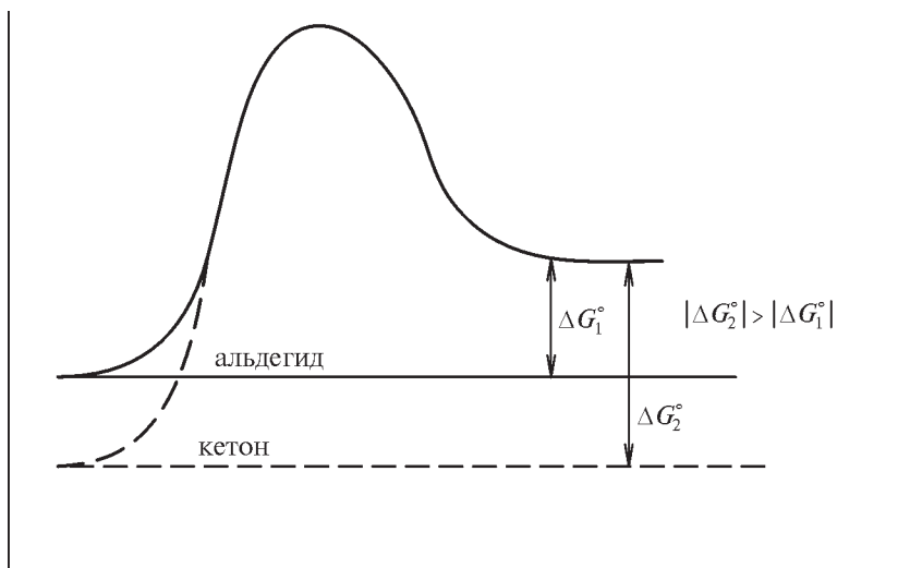
Рис. 16.1. Энергетическая диаграмма для обратимого присоединения нуклеофильного агента NuH к альдегидам и кетонам
