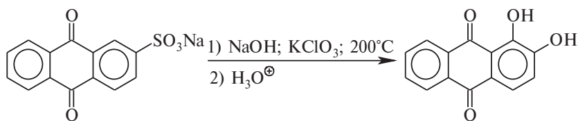
ализарин (1,2-дигидроксиантрахинон)
