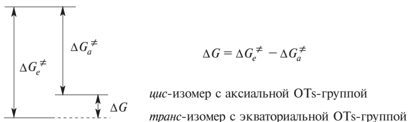
Рис. 22.4. Соотношение энергий активации сольволиза цис - и транс -изомеров тозилатов 4- трет -бутилциклогексанола соответственно с аксиальной и экваториальной тозилокси группой
