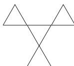
3-ротан
