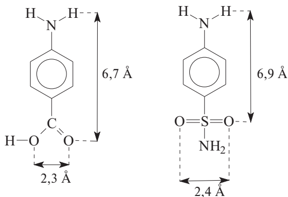
Рис. 19.1. Структурное подобие para -аминобензойной кислоты и сульфаниламида
