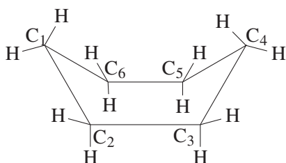
конформация ванны
