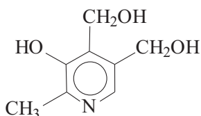
пиридоксин (витамин B 6 )
