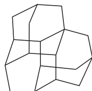
триамантан
