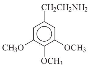
мескалин
