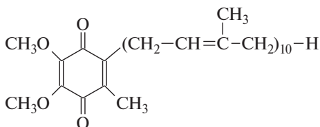
убихинон (коэнзим Q 10 )
