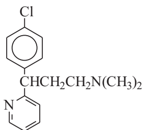
хлорфенирамин
