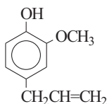
4-аллил-2-метоксифенол, (эвгенол)
