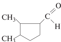
2, 3-диметилциклопентанкарбальдегид
