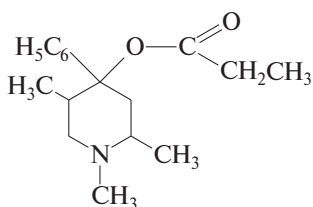
промедол
