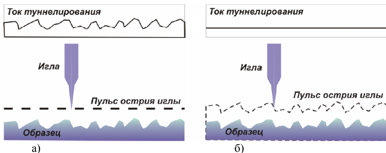
Рис. 14. Режимы работы СТМ: а) изменяющийся туннельный ток; б) постоянный туннельный ток.
