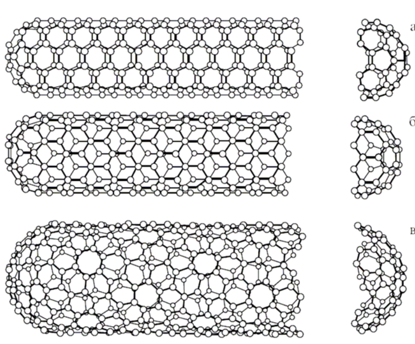
Рис. 36. Примеры возможных структур нанотрубок, зависящих от способа сворачивания графитового листа: а – кресельная структура; б – зигзагообразная структура; в – хиральная структура [59].
