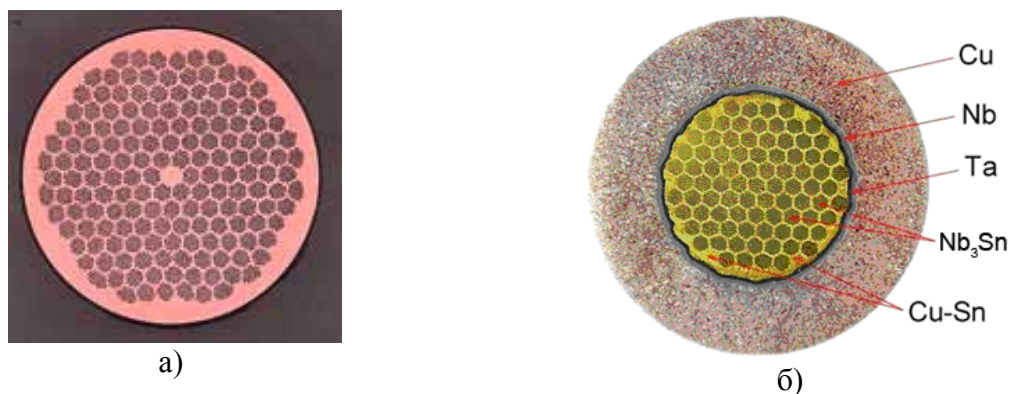
Рис. 27. Сверхпроводящие наноструктурированные материалы для термоядерной энергетики [44].
