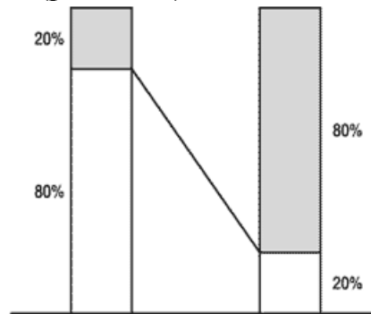
Рис. 2.19. Закон «80/20»
