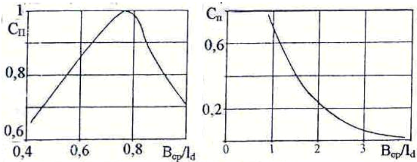
Рисунок2.2- Зміна коефіцієнта C_n під впливом ширини розкату ( V_{cp}/l_d ) при m < 50
