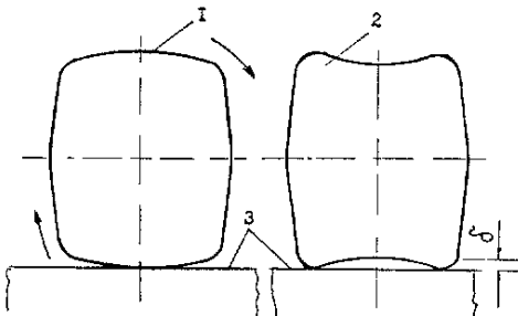
Рисунок 1.6-Розкат після прокатки в ящичному калібрі і кантування : 1-з початковим плоским, але зношеним, дном; 2 - з опуклим дном; 3 - ролик рольганга
