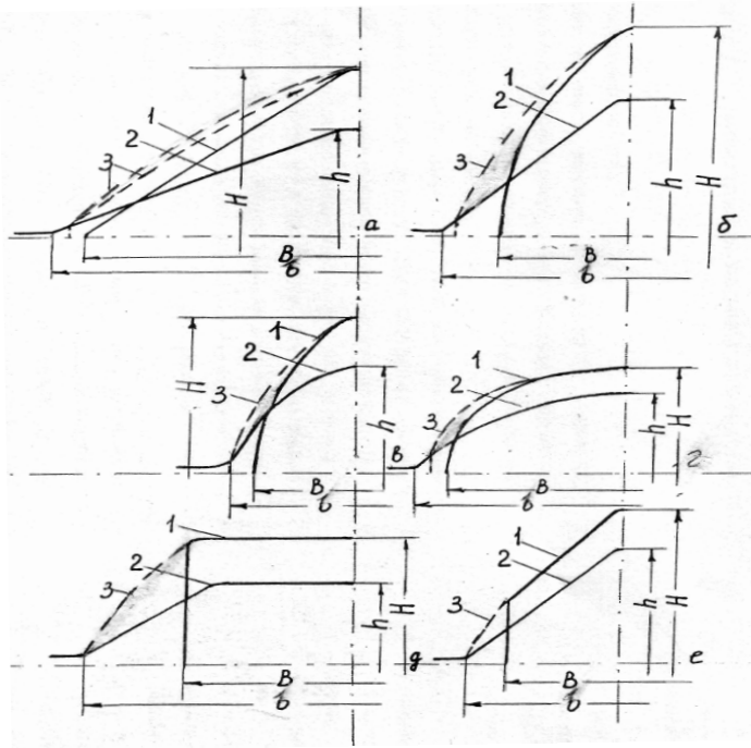
Рис.1.19. Системи калібрів : а - ромб-квадрат; б - овал-квадрат; в - овал - ребровий овал; г - ребровий овал-овал; д - квадрат-шестикутник; е - шестикутник-квадрат (1 - контур заготовки; 2 - калібр; 3 - контур обтиснення заготовки))
