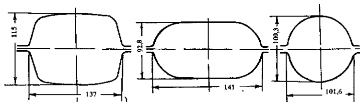
Рисунок 4.4- Система калібрів : підготовчий прямокутник – овал - круг
