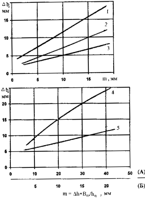
Рисунок 2.3-Розширення по осі калібрів різних форм при прокатки: 1 - овал-квадрат; 2 - ромб-квадрат (квадрат-ромб); 3 - ромб-ромб; 4 (А) - квадрат-овал (овал-квадрат); 5 (Б) - круг-овал (овал-круг). Шкала А - для кривої 4; шкала Б - для кривої 5. (Дані Г. Цоухара при C_{\text{II}}=0,8 )
