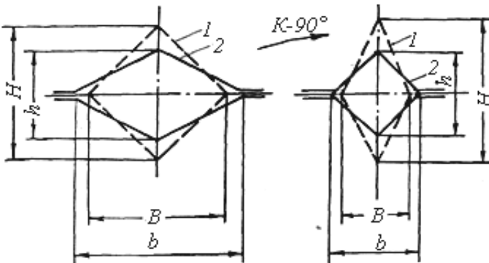
Рисунок 1.12- Система калібрів ромб – квадрат
