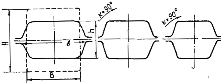
Рисунок 1.8- Ящична система калібрів
