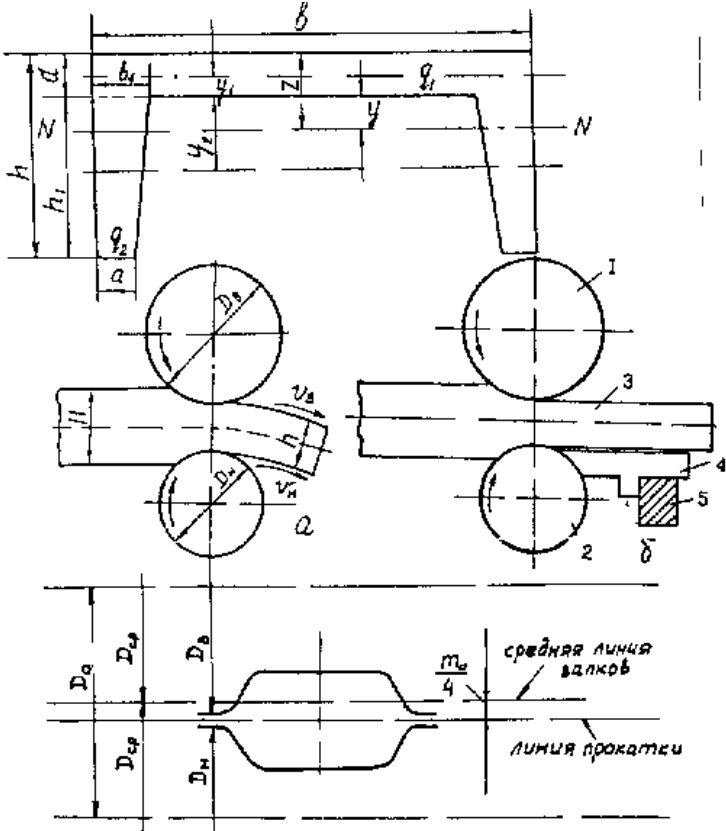
Рисунок 1.20- Швелерний калібр
