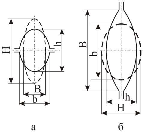
Рисунок 1.13- Система калібрів: а - овал - ребровий овал; б – ребровий овал-овал
