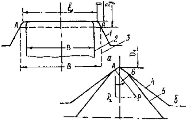
Рисунок 3.1 - Схема захвату прямокутного розкату в ящичному калібрі (а) і ромбічного розкату в квадратному калібрі (б) : 1, 4 - контур калібру; 2 - розкат при B < b_d ; 3 - розкат при B > b_d ; 5 - контур ромбічної заготовки
