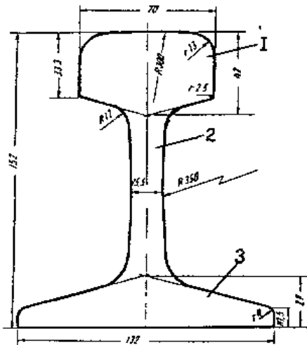
Рисунок 4.5- Профіль рейки Р-50: 1 - головка; 2 - шийка; 3 - підшва
