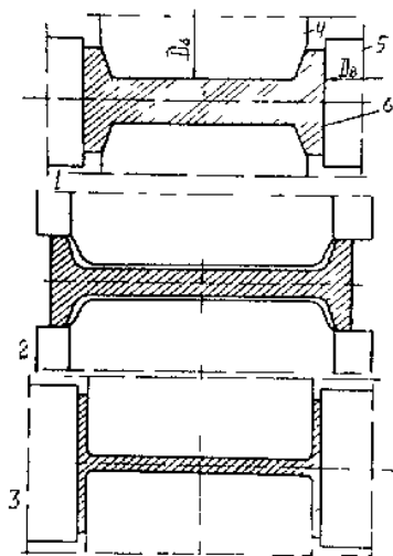
Рисунок 4.12 Схема розташування валків для прокатки широкополочних балок : 1 - чорнова універсальна кліть; 2 - допоміжна кліть; 3 - чистова універсальна кліть; 4 - горизонтальні валки; 5 - вертикальні валки; 6 - розкат балки
