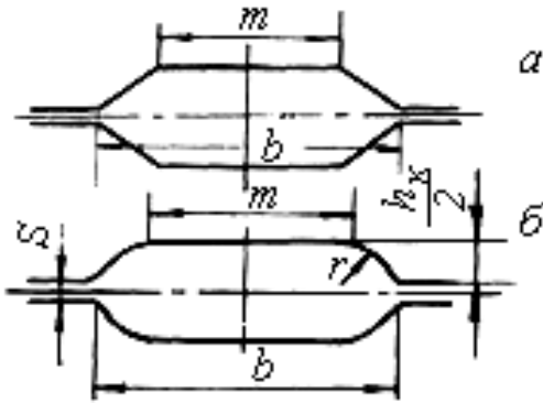
Рисунок 1.11. Калібри: а - шестикутник; б - плоский овал
