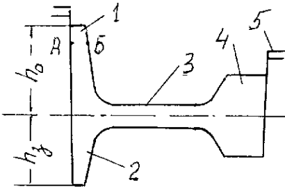
Рисунок 4.8-Рейковий калібр: 1 - відкритий фланець; 2 - закритий фланець; 3 - шийка; 4 - головка; 5 - проміжок між валками
