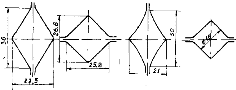
Рисунок 4.15- Передчистовий і чистовий калібр системи ромб - квадрат
