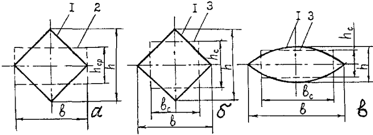
Рисунок 1.18- Форми профілів (1) приведеного (2) і відповідного (3)
