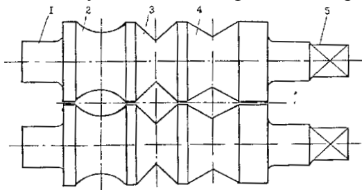
Рисунок 1.1- Валки сортового стана : 1-шейка; 2-4 - калібри; 5 - хвостовик
