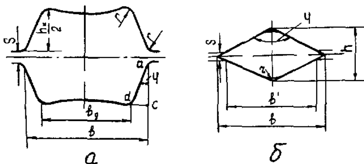
Рисунок 1.3- Ящичний (а) і ромбічний (б) калібри
