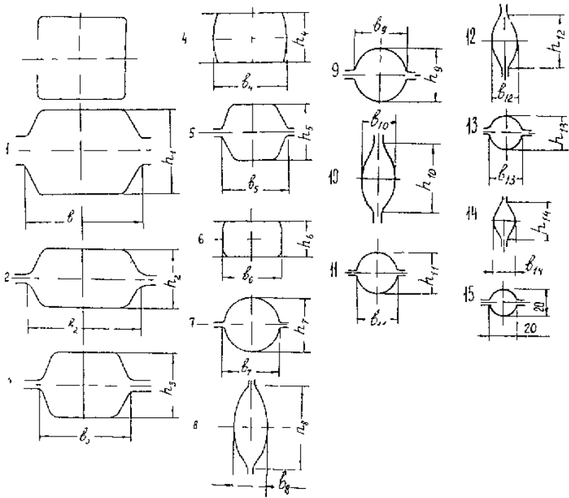
Рисунок 4.14-Схема калібрування валків неперервного дрібносортового стана (I - XV - номери клітей). Прокатка круглого профілю
