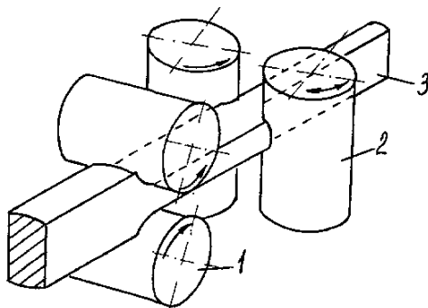
Рисунок 1.16- Прокатка в системі гладка бочка - гладка бочка: 1 – горизонтальні валки; 2 - вертикальні валки; 3 - розкат.
