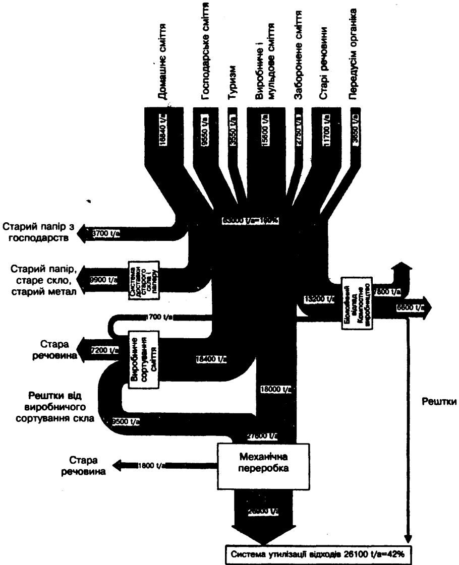
Рис. 5.10. Концепція обробки відходів округу Гарміш-Портенкірхен у ФРН (т/а тоннобіг в рік) (всі показники заокруглені; за Succor, Wittig, 1993).
