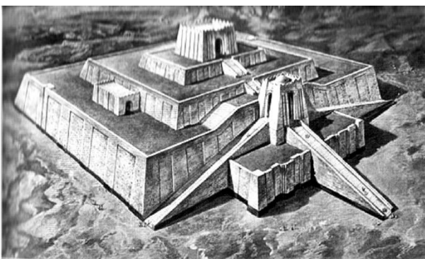
Рисунок 1.1 – Зиккурат Етеменнігуру в Урі (розмір 64x46 м, висота до 30 м)
