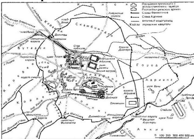
Рисунок 1.6 – План території Афінів та Афінівський Акрополь
