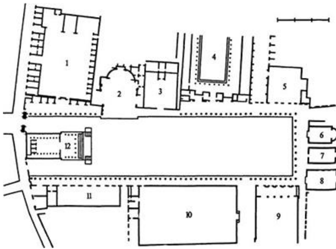
Рисунок 1.10 – План Головного форуму Помпеї
