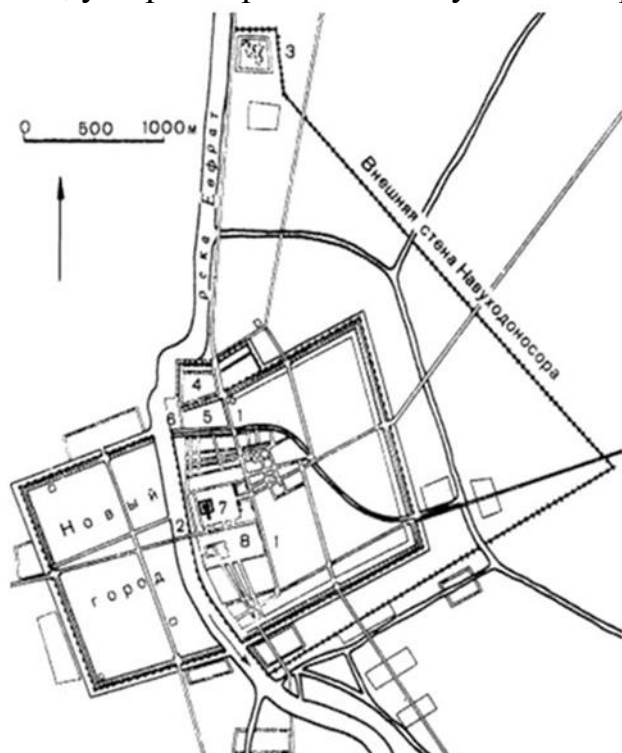
Рисунок 1.2 – Вавилон, план міста у VI ст. до н.е.
