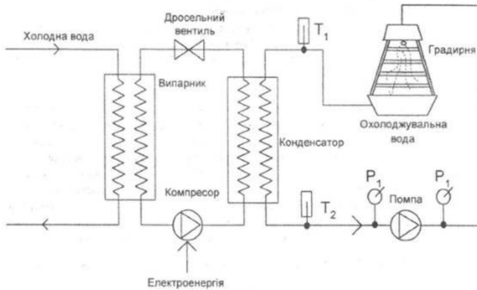
Рисунок 2.8 - Схема холодильної парокомпресорної установки
