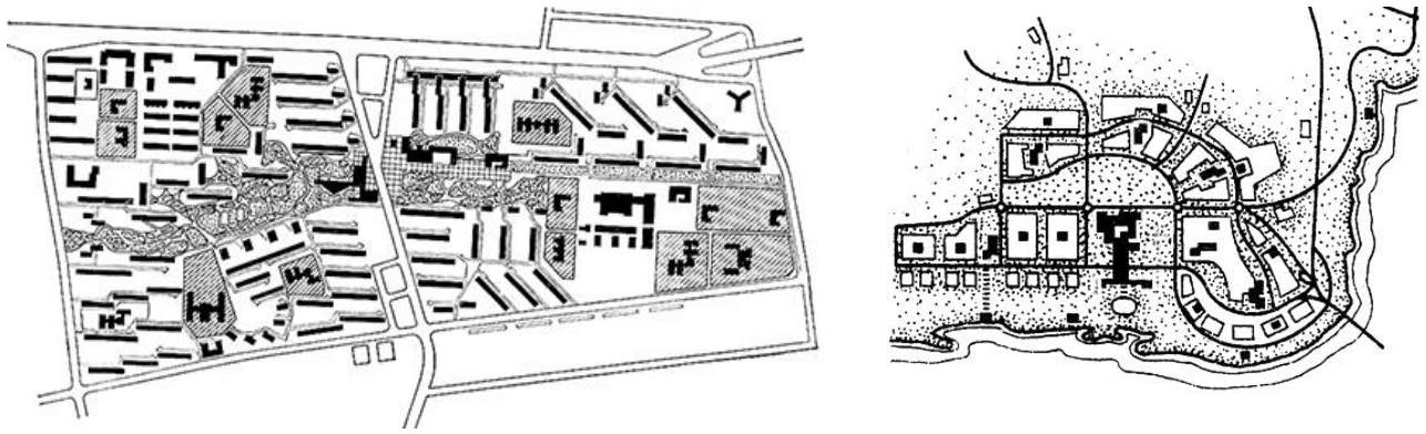
Рисунок 6.2 – Планувальна модель розміщення громадських центрів і установ обслуговування в середніх і великих містах
