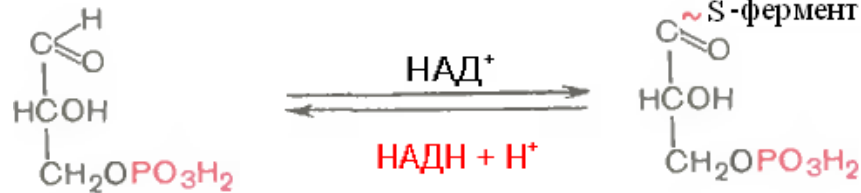
Глицеральдегид-3-фосфат
