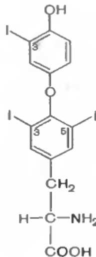
L-3,5,3'-трийодтиронин
