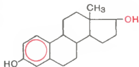
Естрадиол
