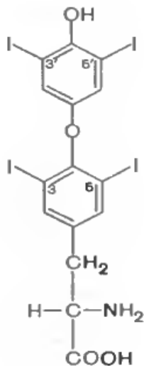
L-тироксин (3,5,3',5'-тетрайодтиронин)
