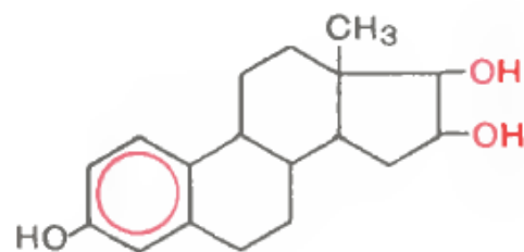
Естриол
