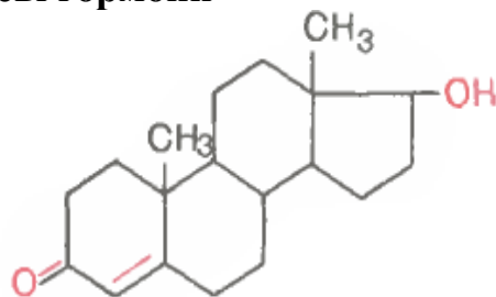
Тестостерон
