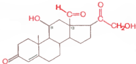
Альдостерон
