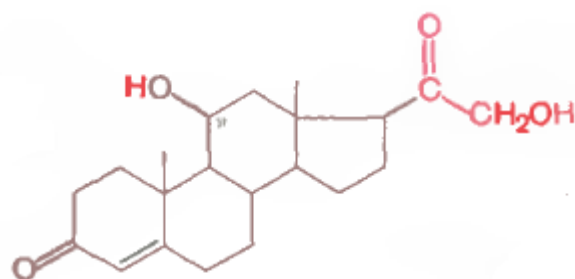
Кортикостерон
