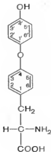
L-тиронин
