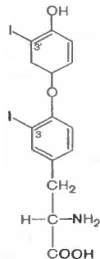
L-3,3'-дйодтиронин
