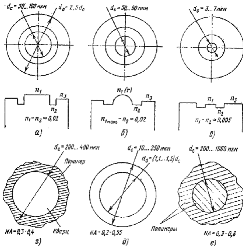
Рисунок 7.3 - Геометрія і профіль зміни показника заломлення кварцевих двошарових багатомодових ступінчастих (а), градієнтних (б), одномодових (в) волокон. Геометрія серцевини і числові апертури кварц-полімерних (г), з багатокомпонентних стеклол (д) і полімерних (е) світлопроводів [15]
