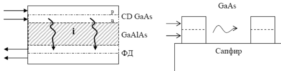
Рисунок 5.4 - Приклади конструкцій оптронів на основі монолітних пристроїв[15]
