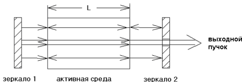
Рисунок 2.5 – Схема пристрою лазера
