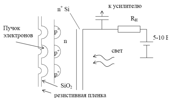
Рисунок 4.2 - Схема пристрою кремнікона[15]
