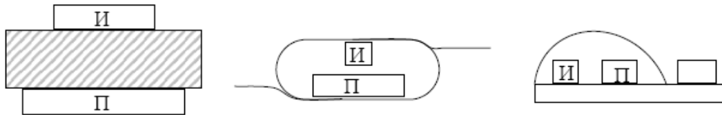
Рисунок 5.2- Прикладів типових конструкцій оптопар[12]
