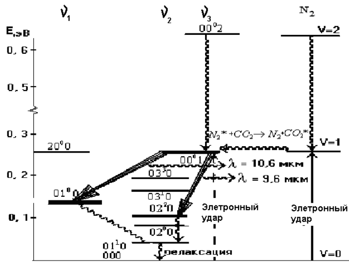
Рисунок 2.14 – Энергетичний спектр молекул CO 2
