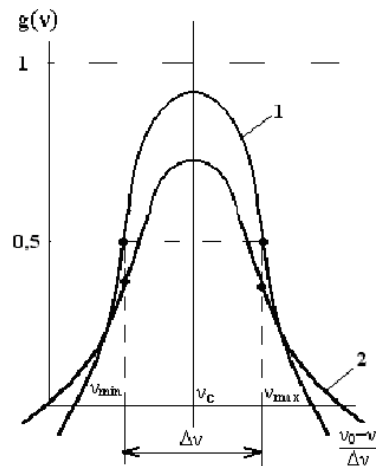
Рисунок 2.8 – Гауссова (1) і Лоренцева (2) форми ліній
