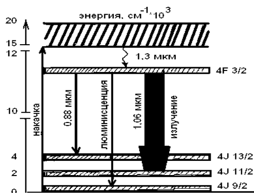
Рисунок 2.16. Діаграма енергетичних рівнів неодима [6]
