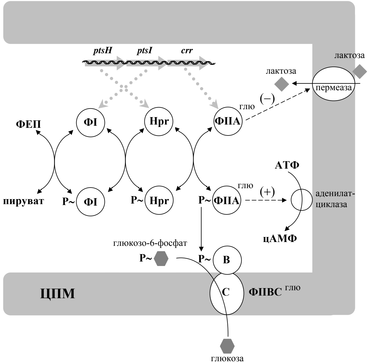
Рис. 2. Схема транспорта ФТС-углеводов и не-ФТС-субстратов в клетки энтеробактерий. Знаками “+” и “-” показано, соответственно, активирующее и ингибирующее действие домена ФП II ГЛЮ .
