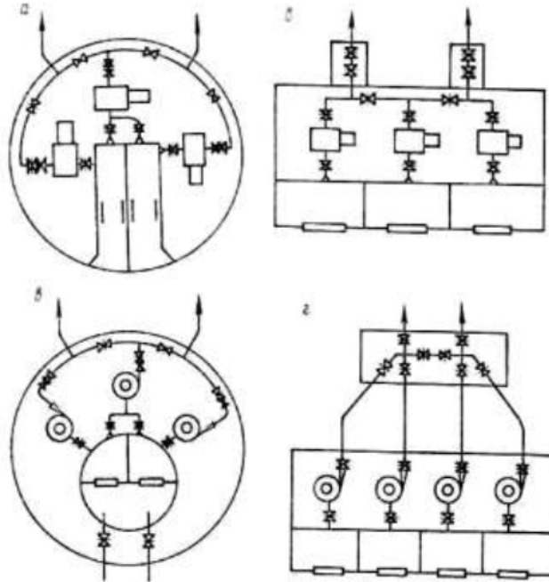
Рисунок 5.3 - Схеми перемикачів усмоктувальних і напірних трубопроводів станцій першого підйому
