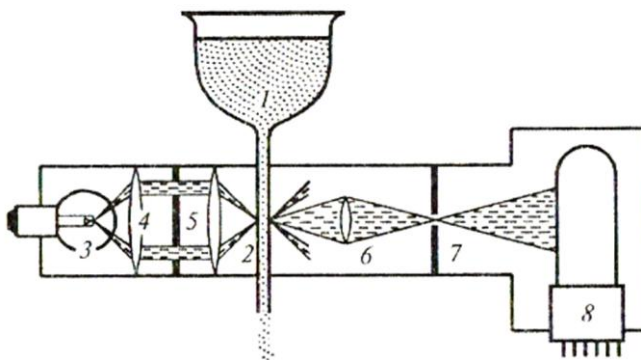
Рис. 6.5. Метод визначення кров'яних клітин на основі мікроскопії темного поля: 1 – розбавлена кров; 2 – тонка трубка; 3 –лампа; 4 – лінза; 5 – діафрагма з кільцевою апертурою; 6 – лінза; 7 – діафрагма; 8 – фотоелектронний підсилювач
