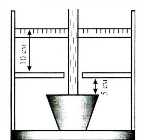
Рис.2.20. Схема приладу для дослідження залежності пружних властивостей ксилеми від впливу механічних стимулів [Hepworth, 1999].
