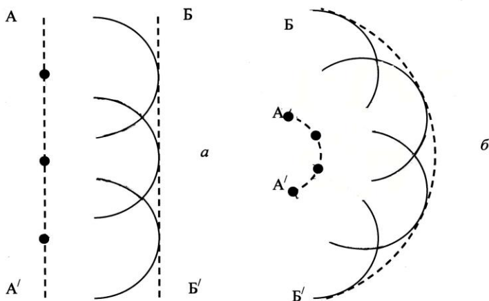
Рис. 23.8. Принцип Гюйгенса: a – плоска хвиля; b – сферична хвиля.
