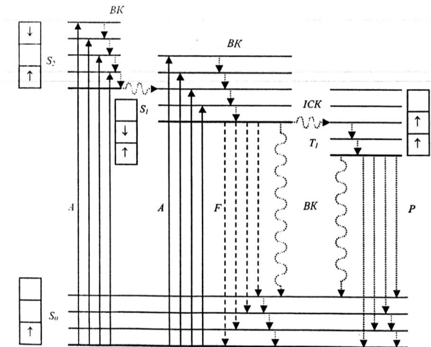
Рис. 24.4. Схема енергетичних рівнів та можливих переходів між ними: S_0 – основний рівень; S_1 , S_2 – синглетні рівні; T_1 – триплетні рівні; КР – ко-
