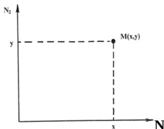
Рис. 8.8. Фазова площина
