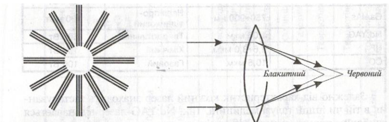
Рис. 22.28. Картина для перевірки наявності астигматизму
