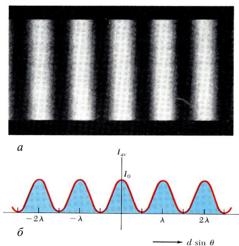
Рис. 23.6. Інтерференція світла: а – інтерференційна картина, б – розподіл інтенсивності світла під час інтерференції (пояснення в тексті)
