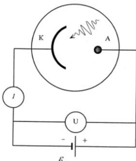
Рис. 23.21. Схема експериментального приладу, за допомогою якого спостерігають явище фотоелектричного ефекту: А – анод, К – катод
