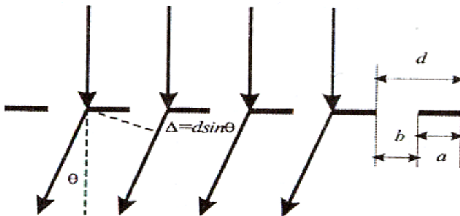
Рис. 23.12. Дифракційна решітка
