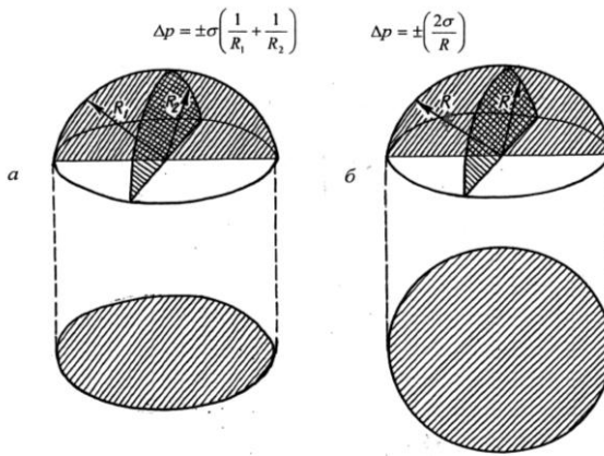
Рис. 5.8. Форма меніска в капілярі: a – еліптична ( R_1 \neq R_2 ); б – сферична поверхні ( R_1 = R_2 = R )
