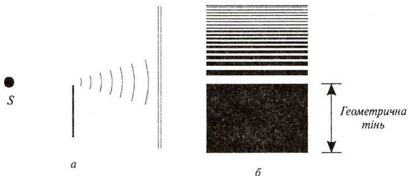
Рис. 23.9. Дифракція світла: a – проходження світла біля різних меж, що супроводжується дифракцією; b – дифракційна картина
