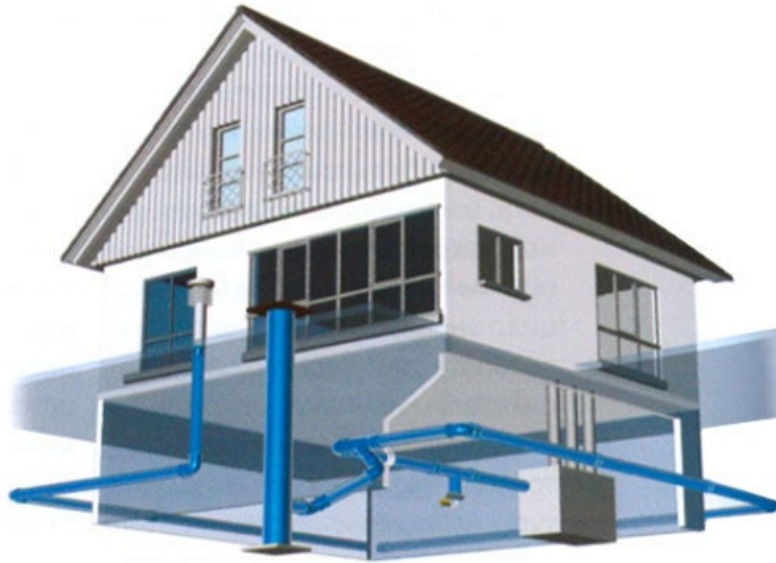
Рисунок 1.9 - Геотермальна схема
