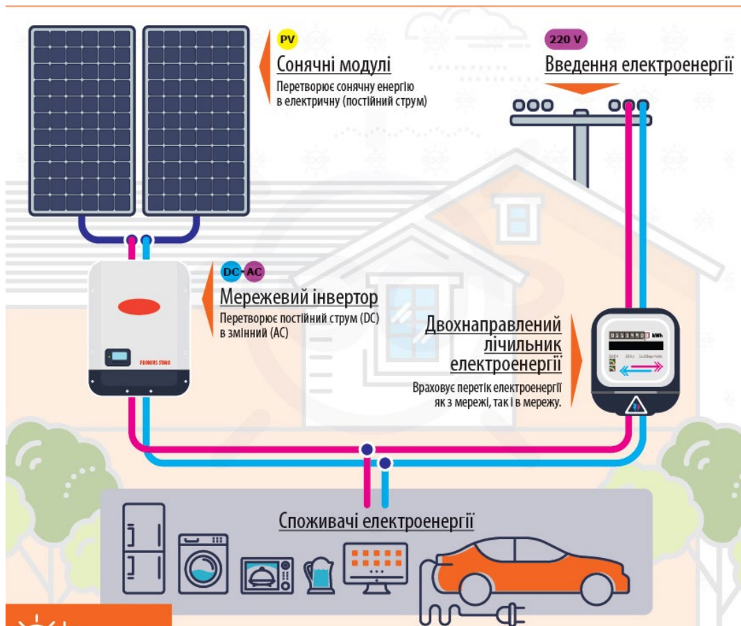
Рисунок 5.3 Схема сонячної електростанції.
