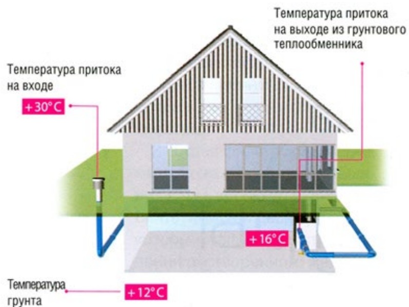
Рисунок 1.10 – Схема роботи підземної вентиляції влітку
