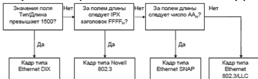
Рис. 3. Алгоритм визначення типу кадру Ethernet
