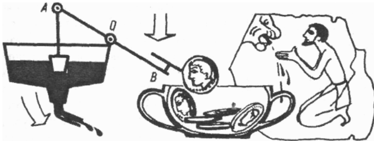
Рис. 3. Перший торговий автомат
