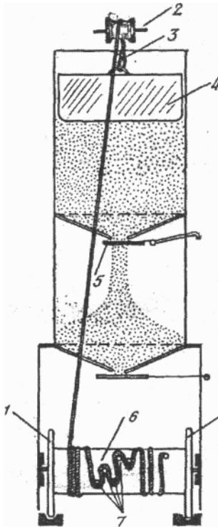
Рис. 5. Механізм автоматичного таксометра: 1 – колеса; 2 – блок; 3 – трос; 4 – тягарець; 5 – заслінка; 6 – барабан; 7 – штирі на барабані.
