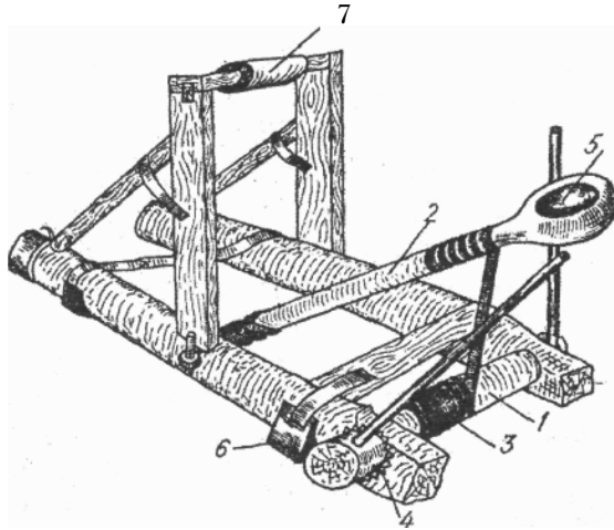
Рис. 2. Стародавня катапульта: 1 – коловорот; 2 – важіль; 3 – пружина; 4 – храповик; 5 – камінь; 6 – засувка храповика; 7 – поперечка.
