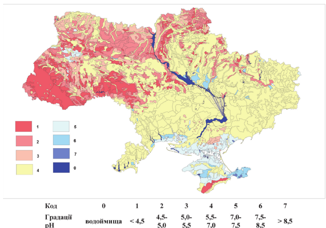
Рис. 1. Кислі ґрунти
