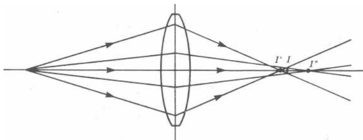
Рис. 4.27. Возникновение сферической aberrации в положительной линзе
