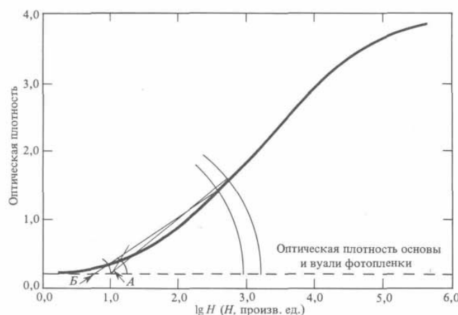
Рис. 8.7. Определение показателя контрастности.
