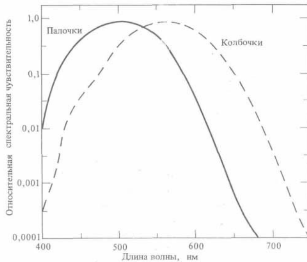
Рис. 6.4. Спектральная чувствительность палочек и колбочек глаза человека
