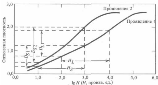
Рис. 8.5. Влияние условий проявления и экспонирования на оптические плотности негативов, полученных при фотографировании одной и той же сцены.
