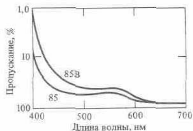
Рис. 13.22. Спектральные кривые пропускания светофильтров № 85 и № 85В
