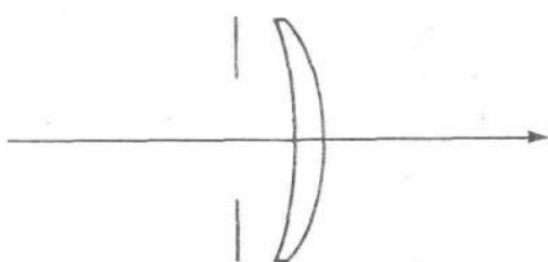
Рис. 4.38. Простейший менисковый объектив Волластона
