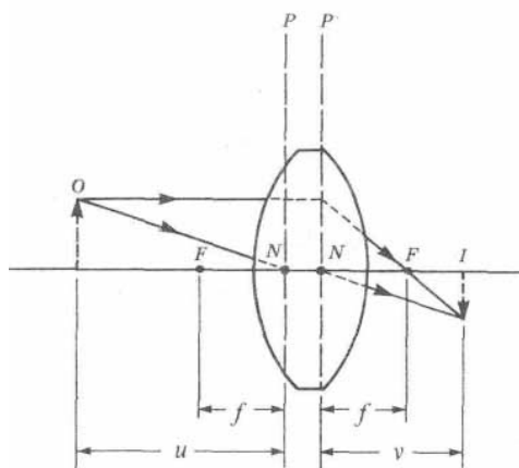
Рис. 4.22. Построение изображения предмета, находящегося на бесконечности, в толстой линзе.
