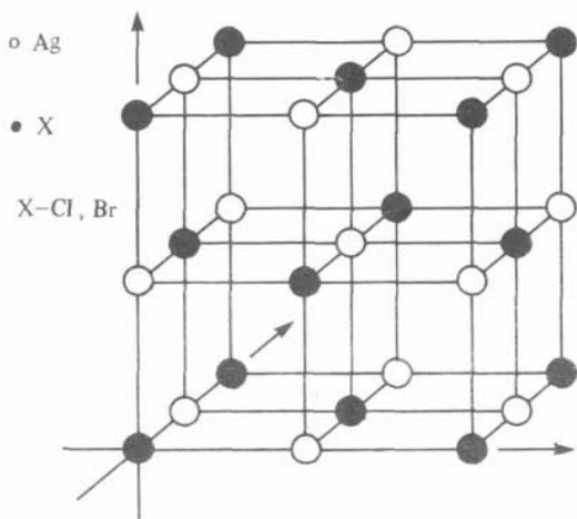
Рис. 7.3. Кристаллическая решетка хлорида и бромида серебра.
