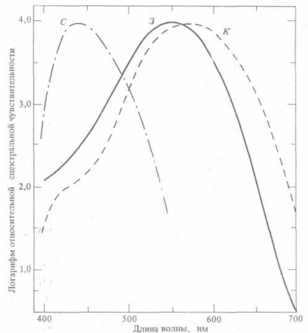
Рис. 6.5. Спектральная чувствительность пигментов трех видов колбочек колбочки, имеющие максимум в средней области длин волн, — зелеными (З) и колбочки с максимумом при больших длинах волн — красными (К). Синие колбочки имеют чувствительность, приблизительно составляющую ОД чувствительности красных и зеленых колбочек. По-видимому, восприятие цвета определяется относительным возбуждением трех типов колбочек. Естественно возникает вопрос о существующих в природе различных типах зрения. Насколько совершенен глаз? Способностью к
