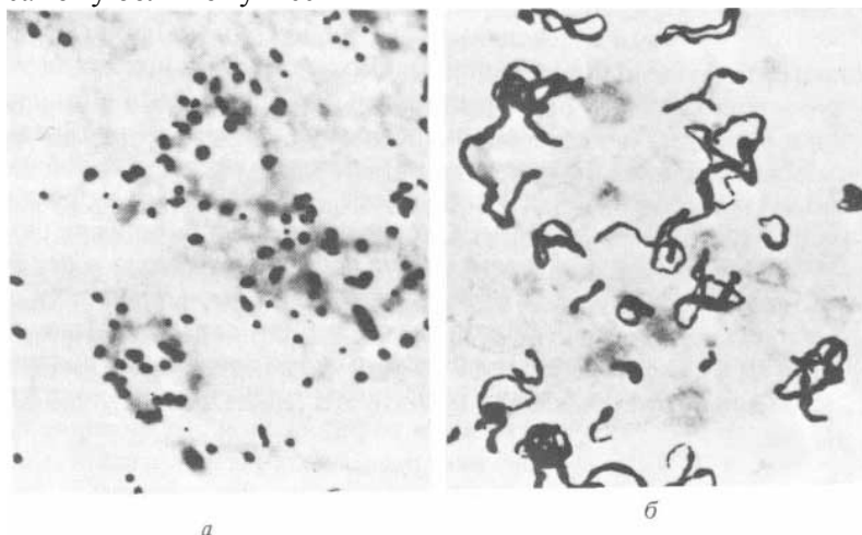
Рис. 7.10. Образование зерен серебра на начальной (а) и конечной (б) стадиях проявления проявителем на основе метола и аскорбиновой кислоты. Из книги В. Carroll, G. Higgins, T. James, Introduction to Photographic Theory, New York: John Wiley, © 1980.
