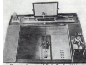
Пишущий телеграф Б. С. Якоби (1841 г.)
