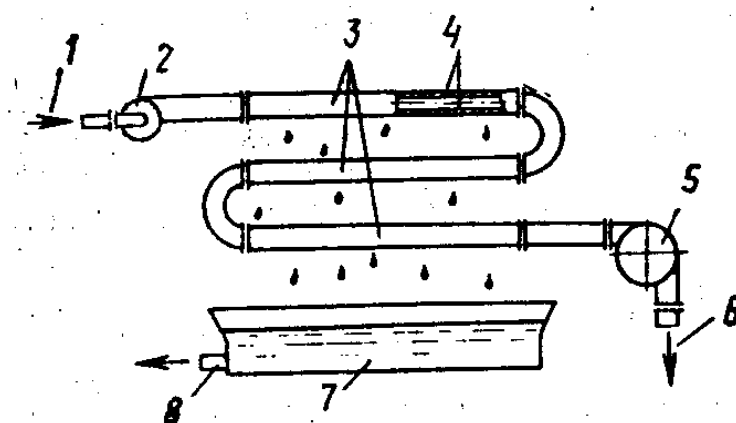
Рисунок 2.31 - Схема трубчастого елементу апарата зворотного осмосу
