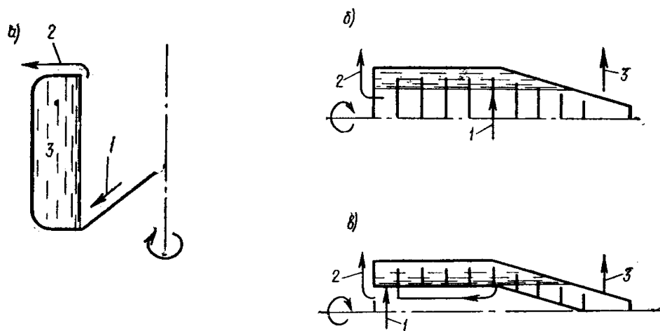
а) маятникова; б) шнекова противоточная; в) шнекова прямоточная. 1 - стічна вода; 2 - фугат; 3 - осад.
