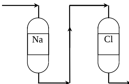
Рисунок 1.6 - Схема установки з натрій-хлор-іонуванням: \text{Na} і \text{Cl} - натрій-катионітовий і хлор-аніонітовий фільтри
