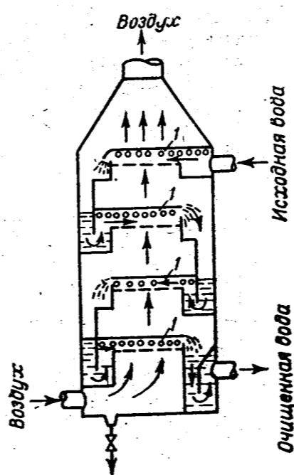
Рисунок 2.29 - Пінний апарат
