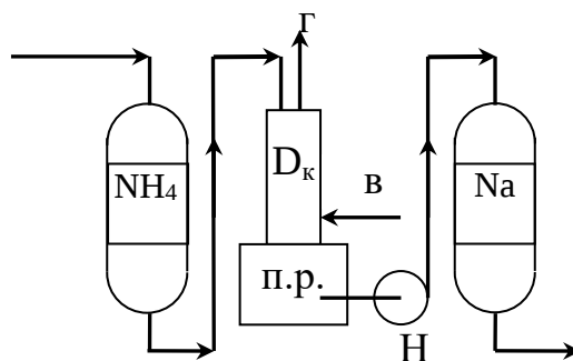
Рисунок 1.5 - Схема установки з амоній-катионітовим фільтром ( \text{NH}_4 ), (позначення див. рис.1.2)
