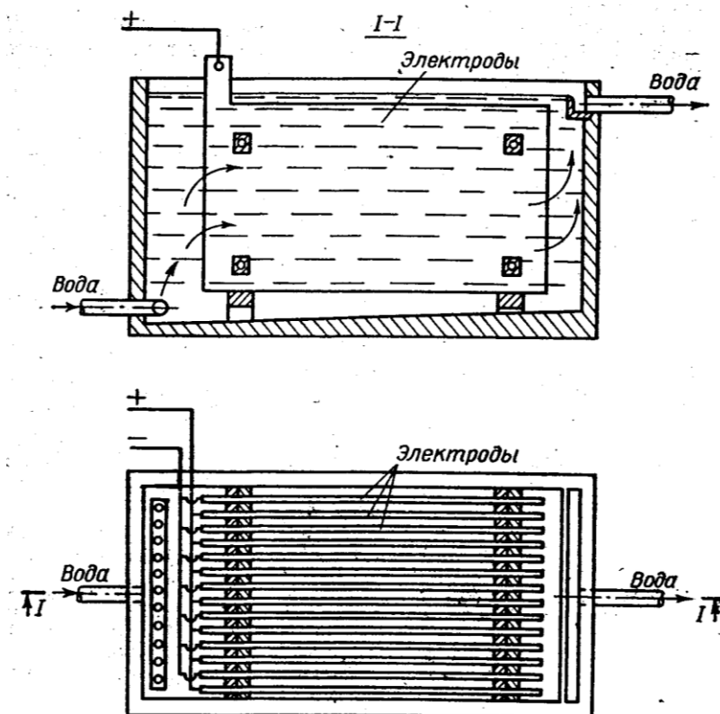
Рисунок 2.20 - Апарат для очистки воды методом электрохимической коагуляции
