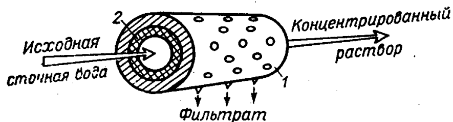
Рисунок 2.31 - Схема трубчастого елементу апарата зворотного осмосу
