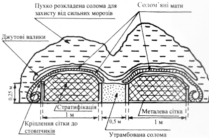
Рис. 23.5. Будова і форма ложа для зимового вермікультування (за Городнім М.М. та ін., 1996)
