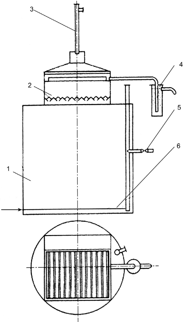
Рис. 22.15. Біореактор для збродження відходів спиртових заводів
