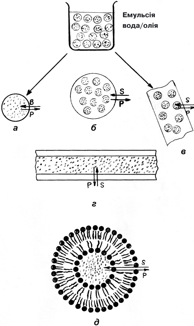
Рис. 7.5. Іммобілізація ферментів з використанням напівпрони- чних оболонок (мембран) (за Березіним І.В. та ін., 1987):
