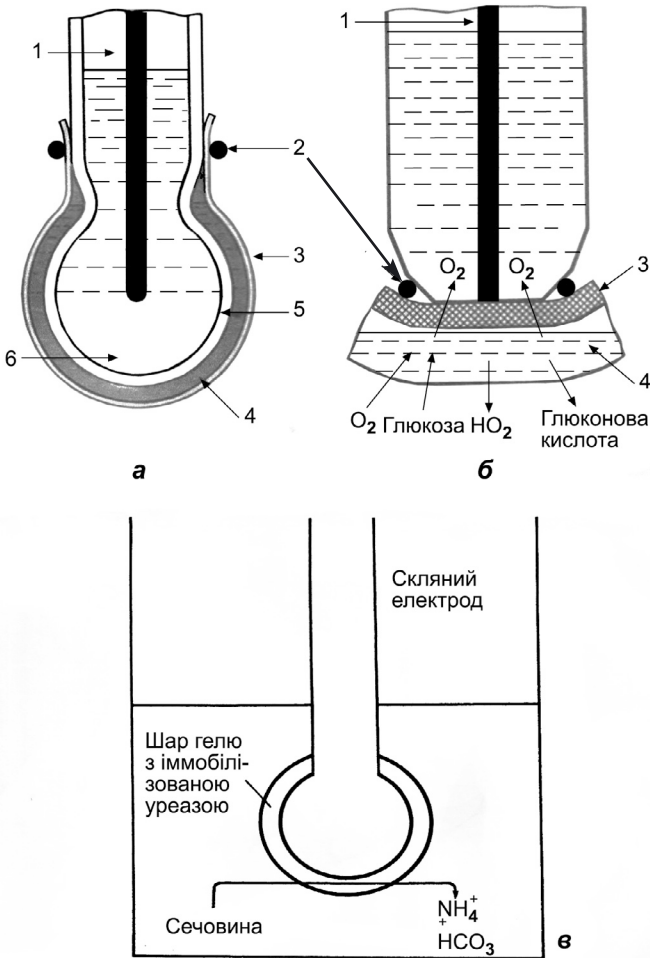
Рис. 9.2. Ферментні електроди (за Березиним та ін., 1987):
