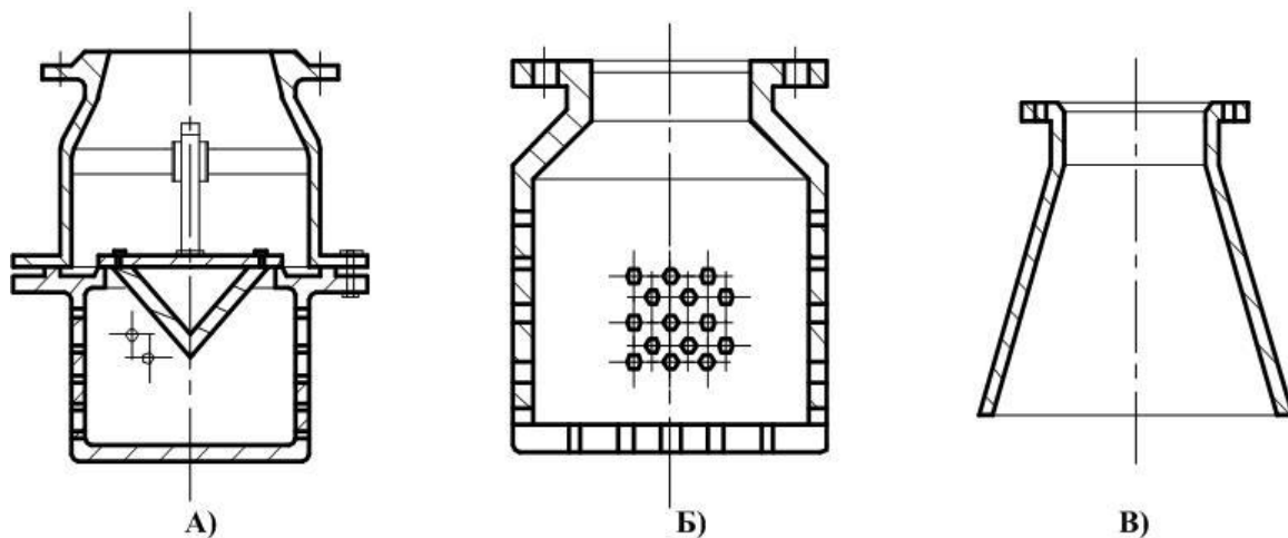
Рисунок 6.1.1 – Приймальне обладнання насосних станцій: А) клапан; Б) сітка; В) лійка
