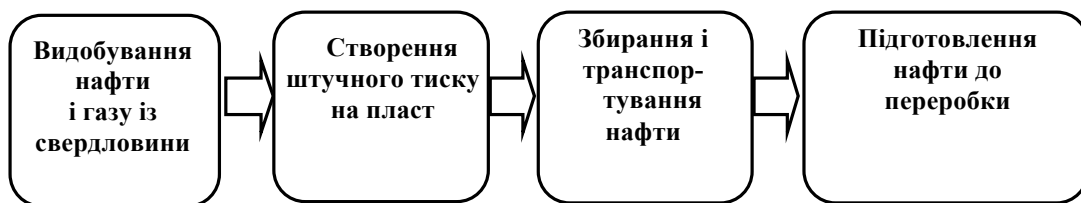
Рис. 3.3. Складові технологічного процесу видобування нафти
