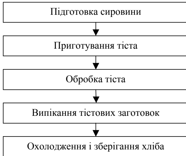
Рис. 9.3. Технологічний процес виробництва хлібобулочних виробів
