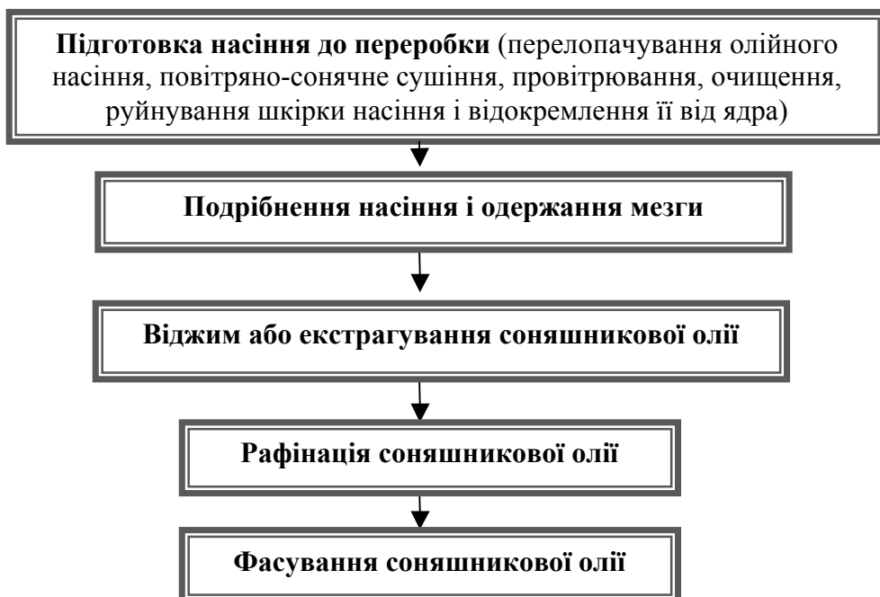
Рис. 9.12. Технологічний процес виробництва соняшникової олії
