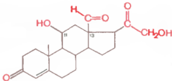
Альдостерон
