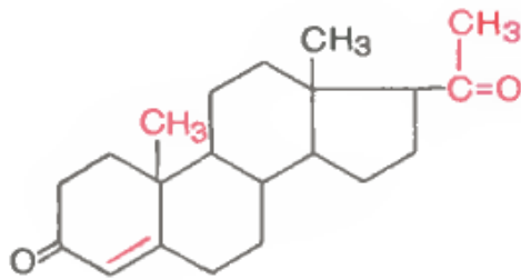
Прогестерон
