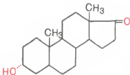
Андростерон
