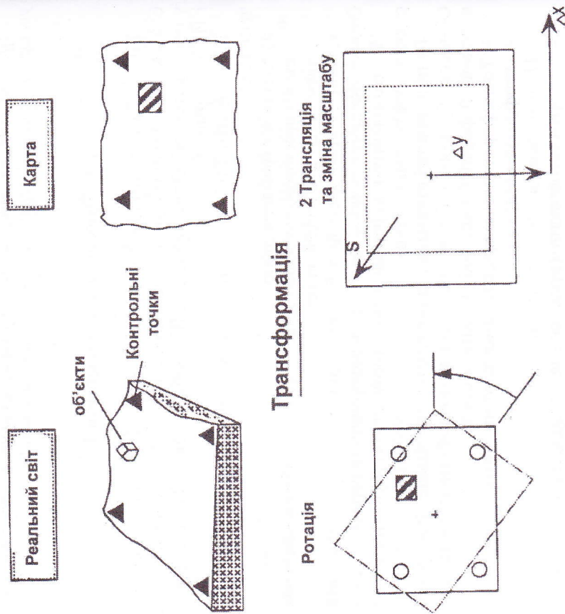
Рис. 1.5. Функція трансформації
