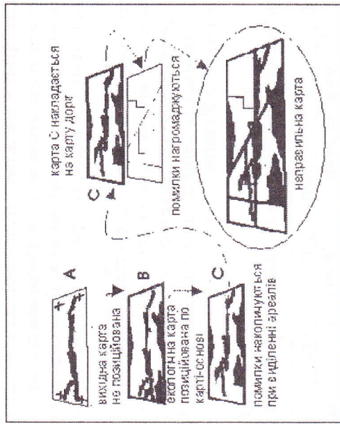
Рис. 5.2. Нагромадження помилок
