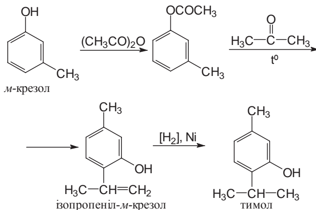
5-Метил-2-(метилетил)фенол
