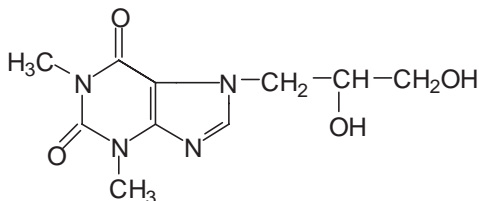
7-(2',3'-Дигідроксипропіл)-теофілін
