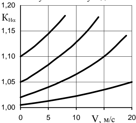
Рисунок Д1 – Коефіцієнт розподілу навантаження між зубамиДодаток
