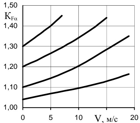
Рисунок Д1 – Коефіцієнт розподілу навантаження між зубамиДодаток
