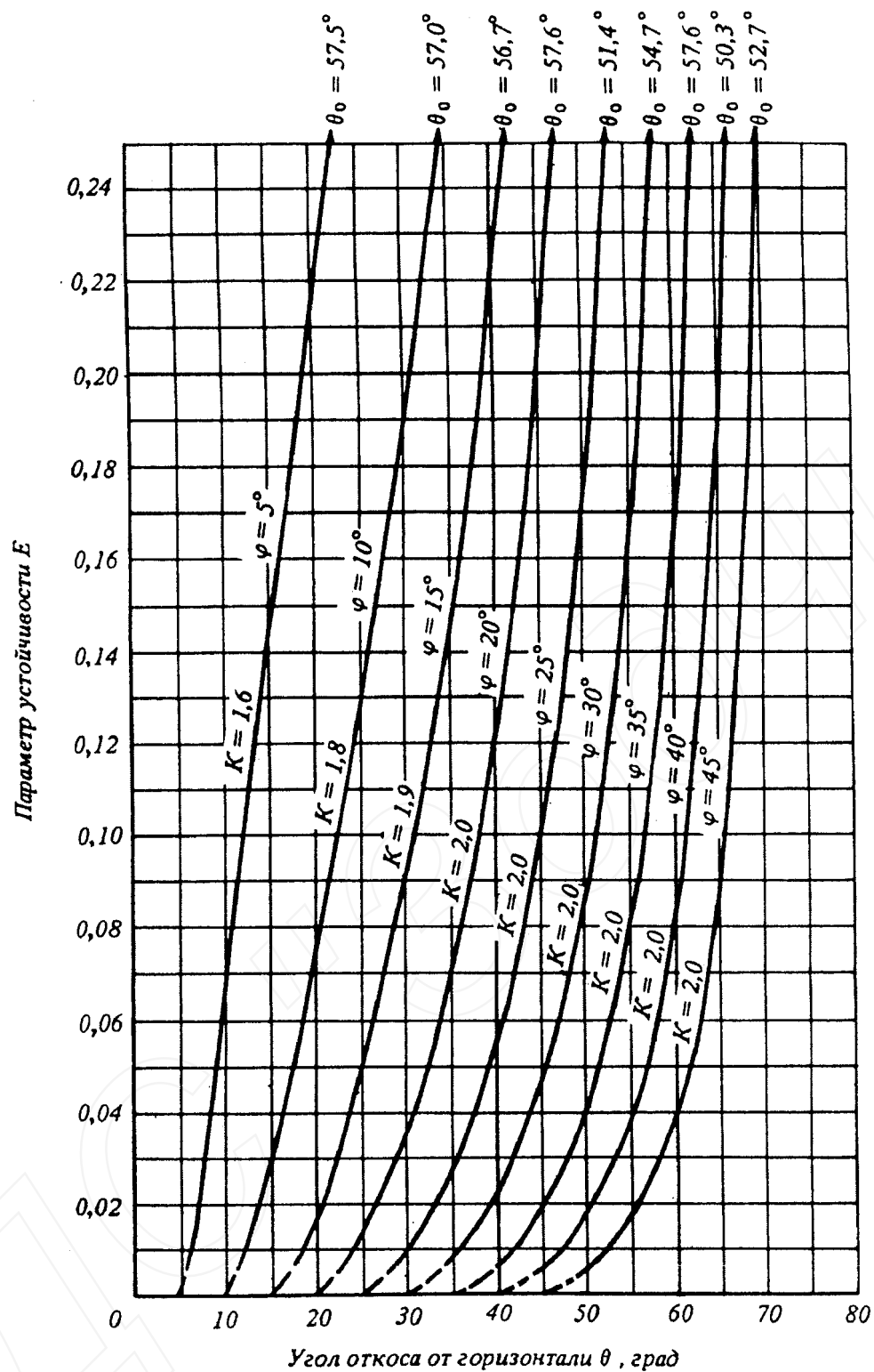
Черт. 3. Графики для определения крутизны откоса при 1 < K \leq 2
