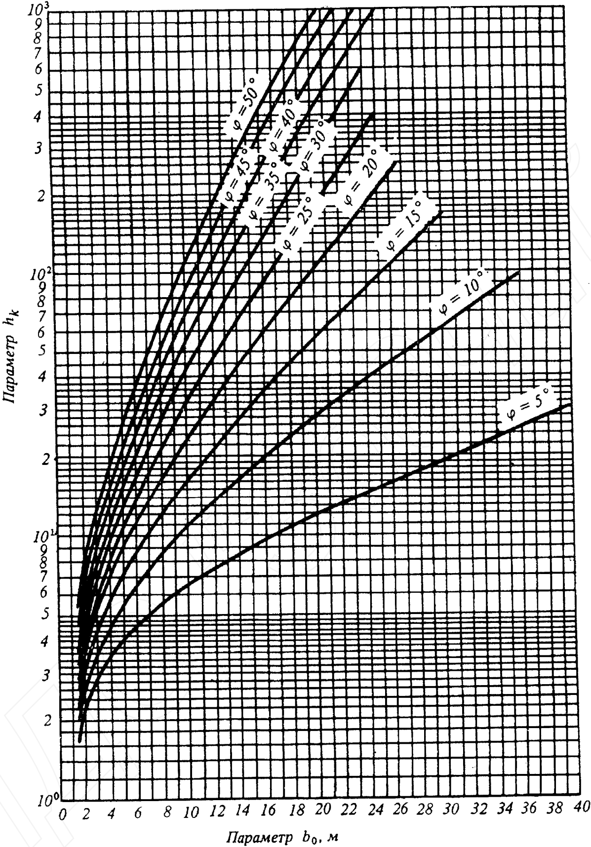
Черт. 6. Графики для определения параметра b_0
