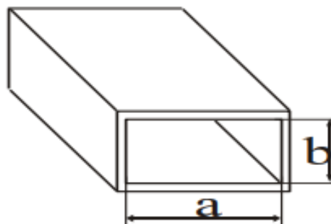
Рисунок - Прямокутний хвилевод
