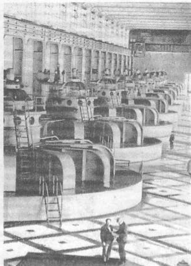
Машинний зал Дніпрогесу після повного відновлення
