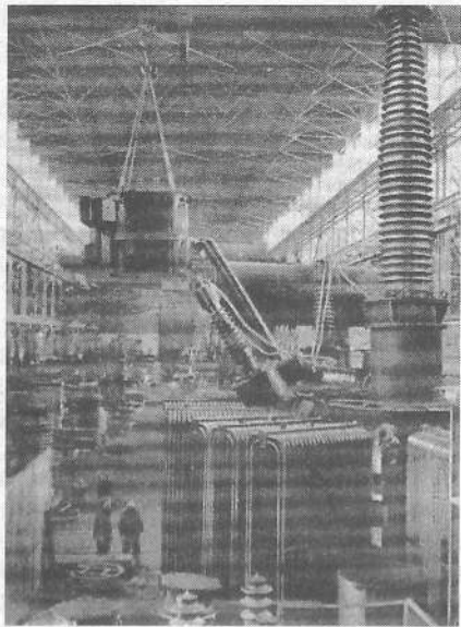
У складальному цеху Запорізького трансформаторного заводу
