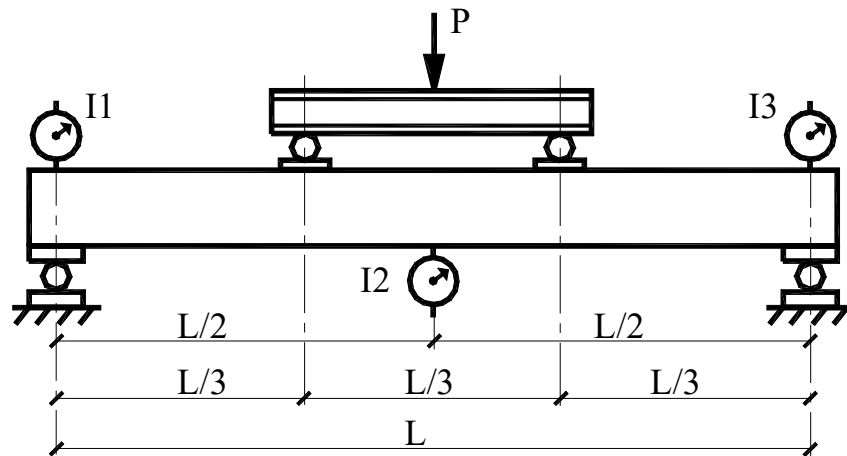
Рис. 2.1. Схема випробування балки та розташування приладів
