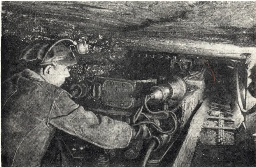
Работа на врубовой машине. Донбасс.
