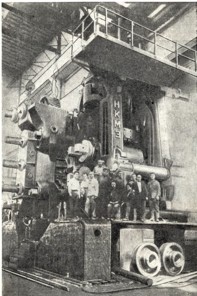
Первый слябинг, изготовленный Краматорским машиностроительным заводом. 1934 г.
