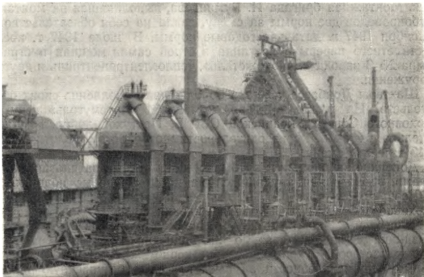
Цельносварная доменная печь завода «Запорожсталь».
