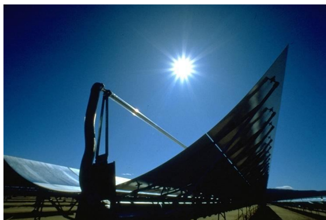
Рис. 7.1. Параболоциліндричний концентратор
