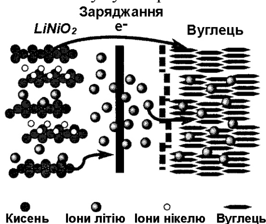
Рис. 2.5. Процес заряджання Li-ion акумулятора
