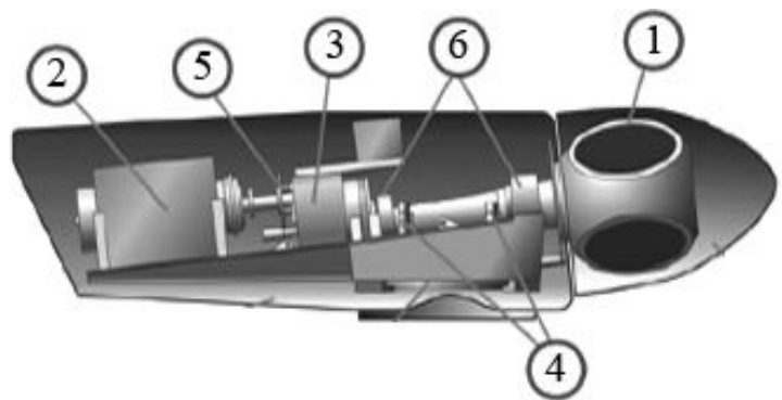
1) втулка вітроколеса; 2) генератор; 3) мультиплікатор; 4) система стеження; 5) гальмо; 6) вал вітроколеса Рис. 8.7. Взаємне розміщення агрегатів у гондолі
