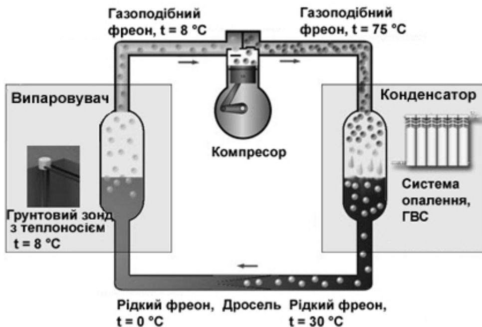
Рис. 5.1. Конструкція ПТН
