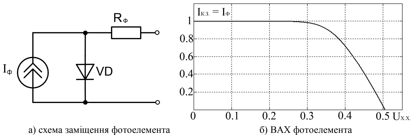
Рис. 7.5. Характеристики фотоелемента
