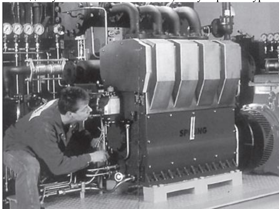
Рис. 4.6. Паровий поршневий двигун
