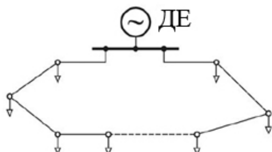
Рис. 9.4. Кільцеві мережі електропостачання
