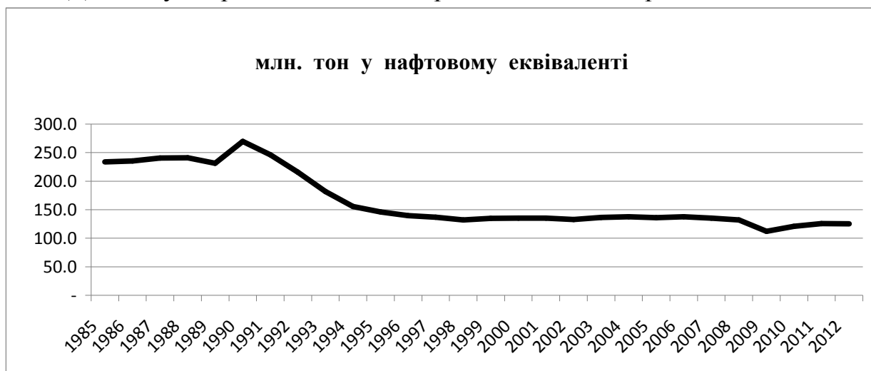
Рис. 1.2. Динаміка енергоспоживання України
