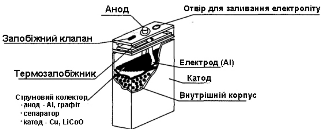
Рис. 2.6. Корпус Li-іон акумулятора
