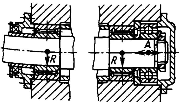
Игольчатые подшипники в комбинации с радиальным шарикоподшипником, разгруженным от внешних радиальных сил и несущим только осевую нагрузку переменного направления
