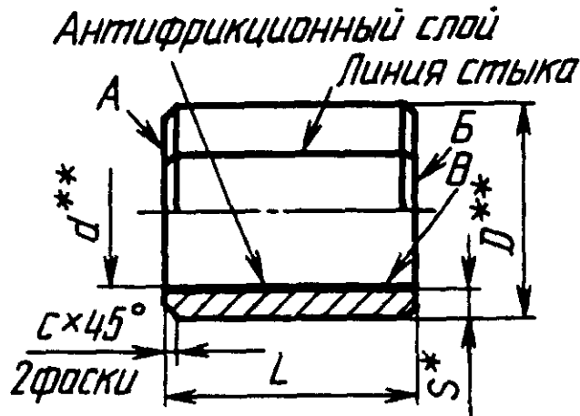
Размеры, мм
