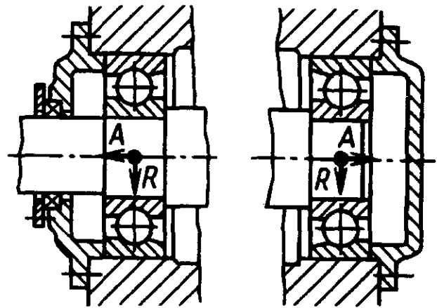
Радиально-упорные шарикоподшипники с узкими торцами наружных колец внутрь в сквозной расточке корпусов, регулируемые набором тонких металлических прокладок между крышками и торцами корпуса
