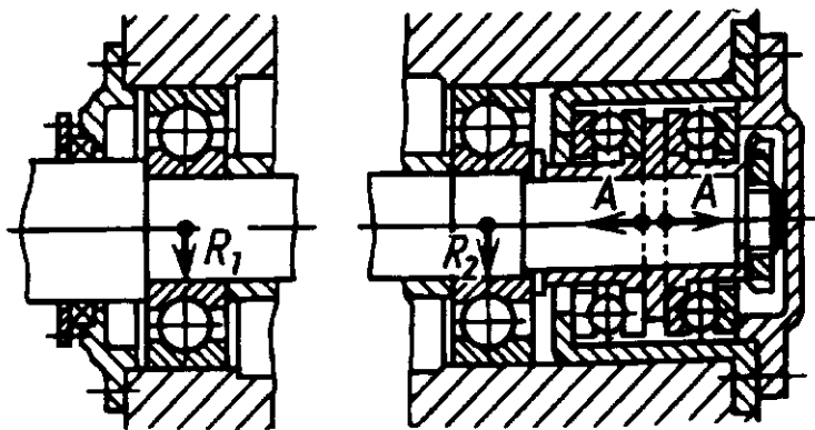
Регулировочные прокладки
