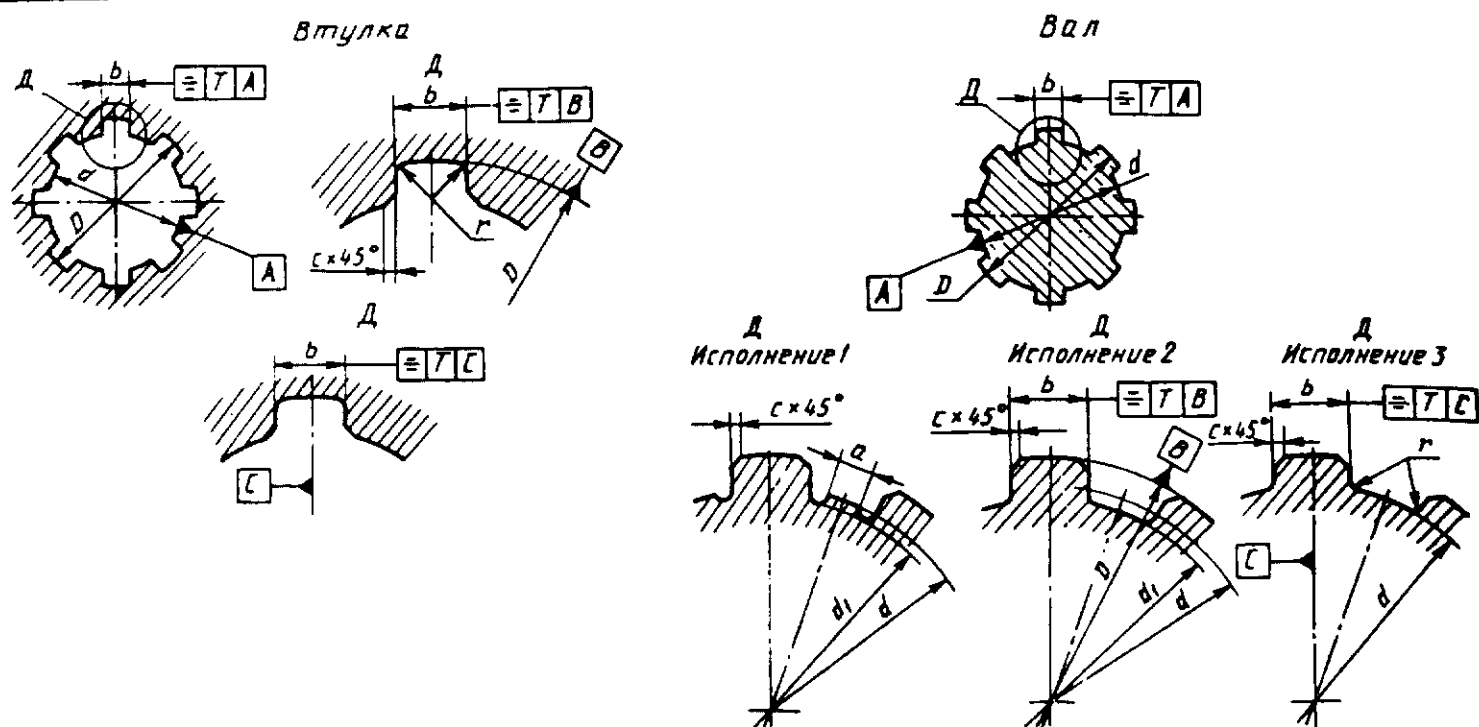
Размеры, мм
