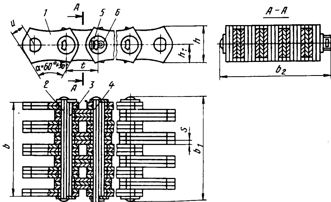
Тип 2
