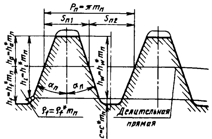
Рис. 35. Исходный контур по ГОСТ 16202-81
