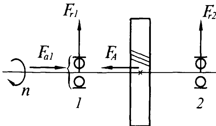
Рис. 28. Расчетная схема к примеру 1
