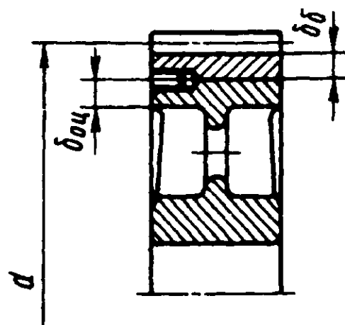
Рис. 23. Конструкция бандажированных цилиндрических колес
