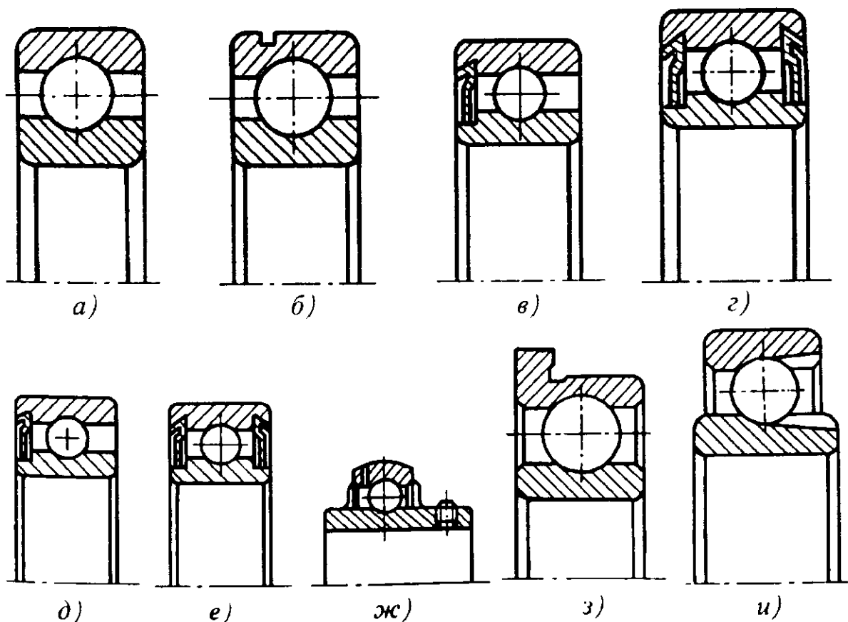
Рис. 13. Подшипники радиальные шариковые исполнений:
