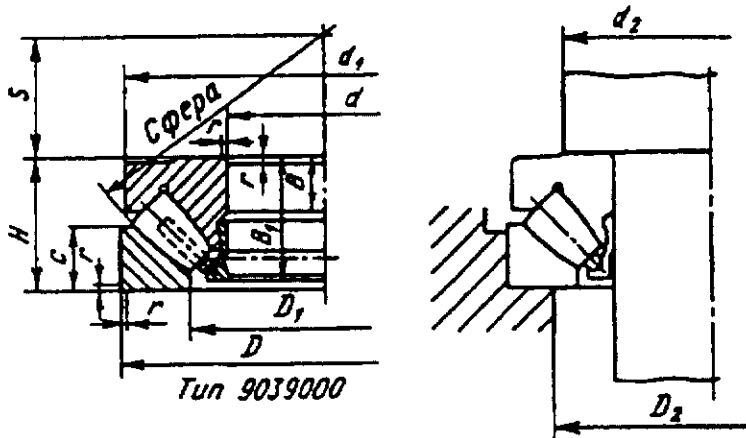
Размеры, мм
