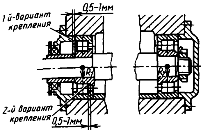
Радиальные роликоподшипники в общей сквозной расточке корпусов
