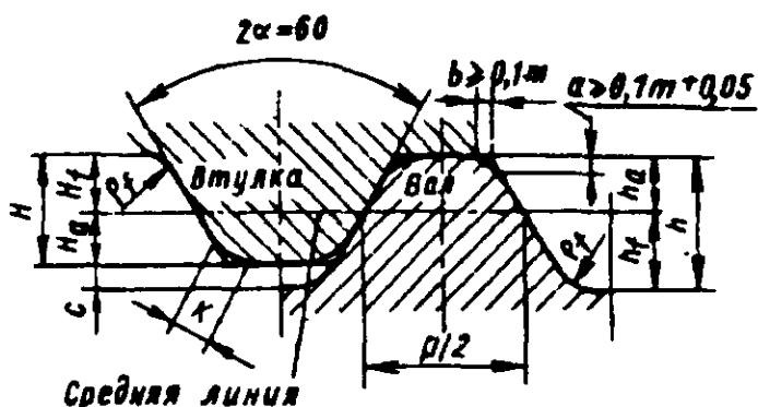
Исходный контур
