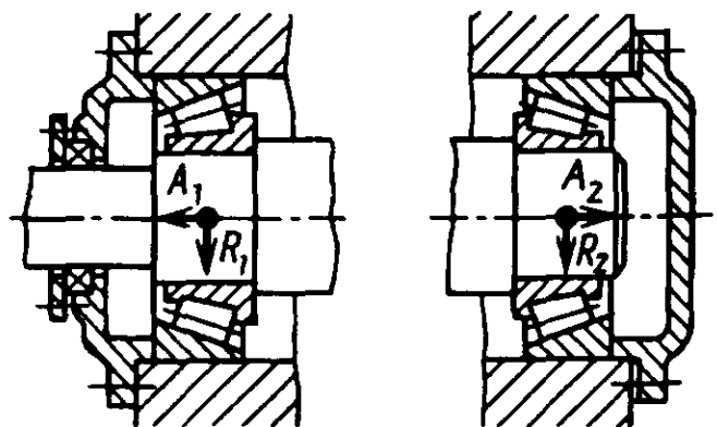
Конические роликоподшипники в сквозной расточке корпусов. Осевая регулировка осуществляется набором металлических прокладок между торцами крышки и корпуса
