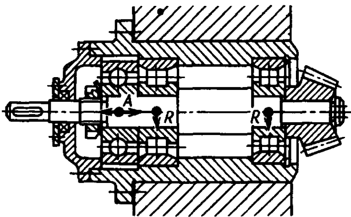
Радиальные роликоподшипники в комбинации с радиальным шарикоподшипником, разгруженным от внешних радиальных сил и несущим только осевую нагрузку переменного направления, в общем стакане
