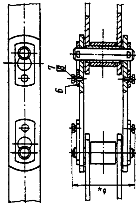
Исполнение 2
