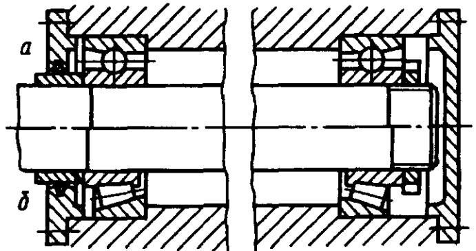
Радиально-упорные подшипники с широкими торцами наружных колец внутрь: а — вариант с шариковыми подшипниками; б — вариант с коническими роликоподшипниками
