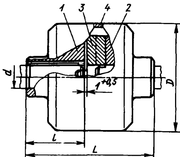
Исполнения 1 и 2
