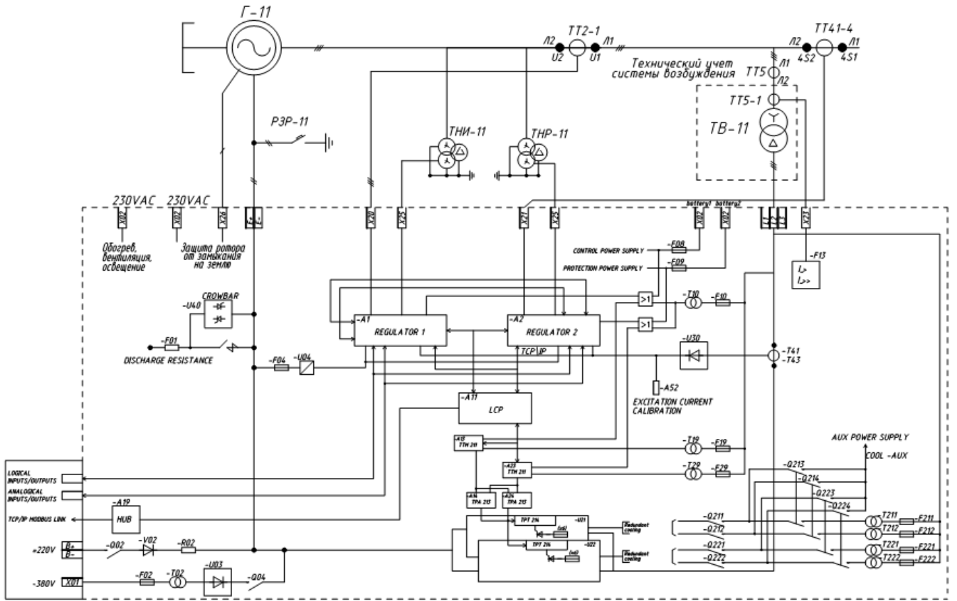
Структурна схема системи збудження гідрогенератора ALSTOM
