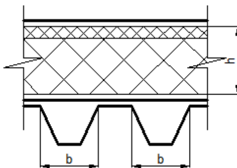
Рисунок 5.8 – Схема розташування утеплювача на проф. настилі
