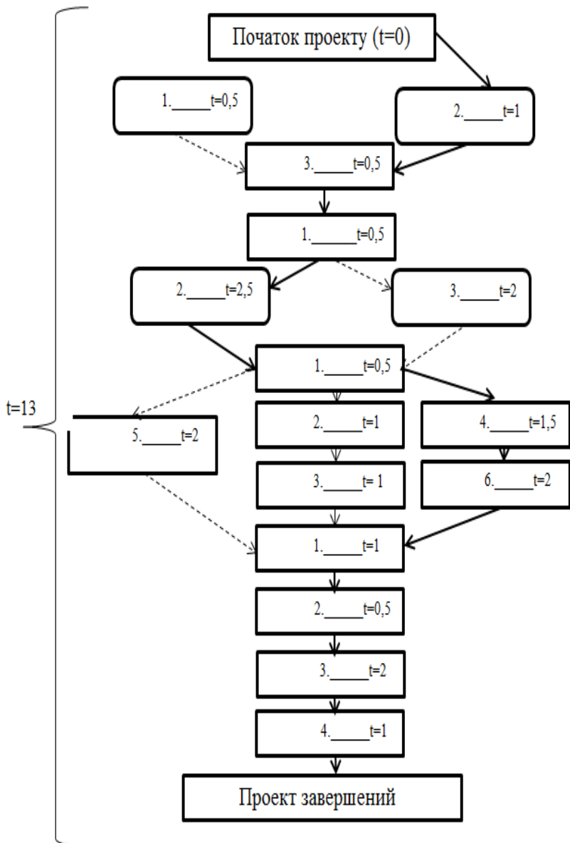
Рис. 2.9. Схема мережевого графіка [21] (критичний шлях зображено суцільними стрілками), [t]=\text{год}
