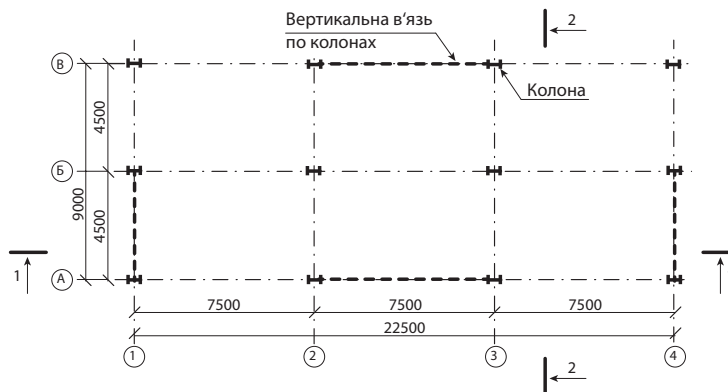
Рисунок 10.1.2 План розміщення колон та вертикальних в'язей у каркасі
