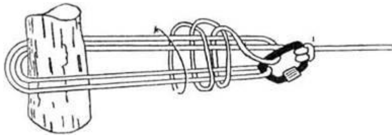
Рис. 4.14. 1 - "напівсхоплюючий" вузол, 2 - вузол "штик".
