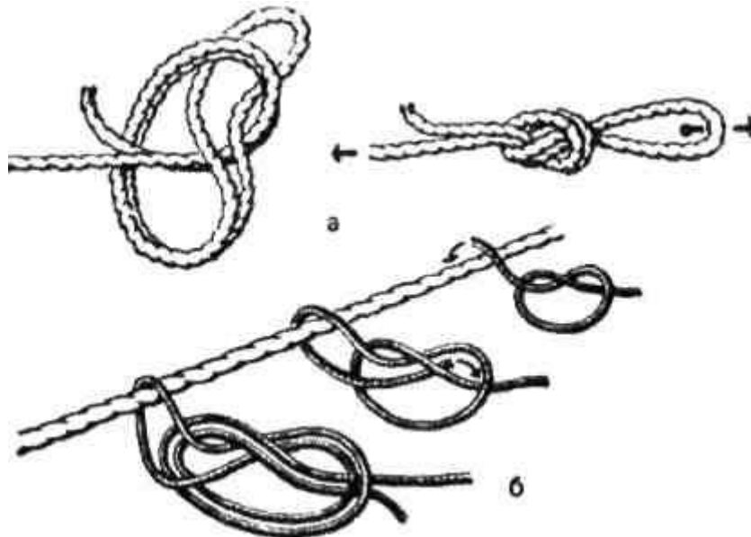
Рис. 3.14. Вузол "провідник": а - в'язання петлею, б - в'язання одним кінцем
