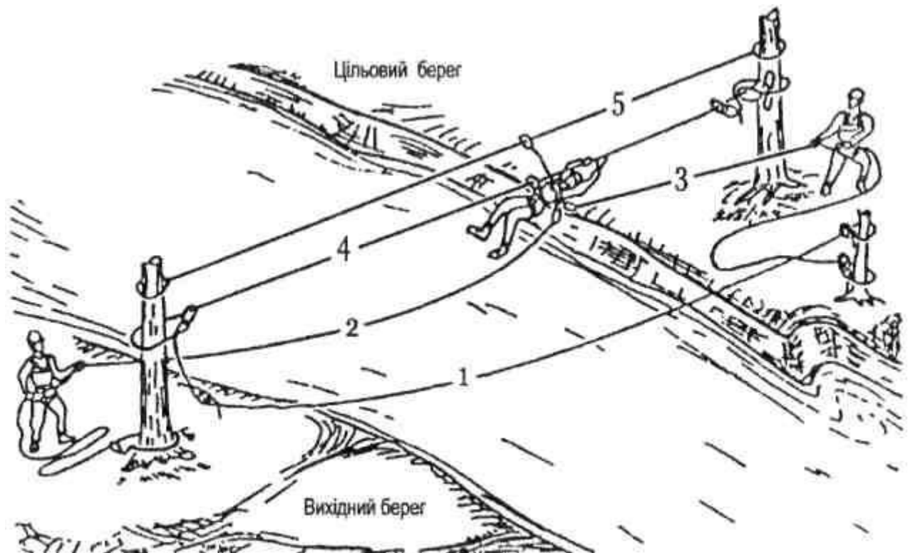
Рис. 4.16. Навісна переправа через річку
