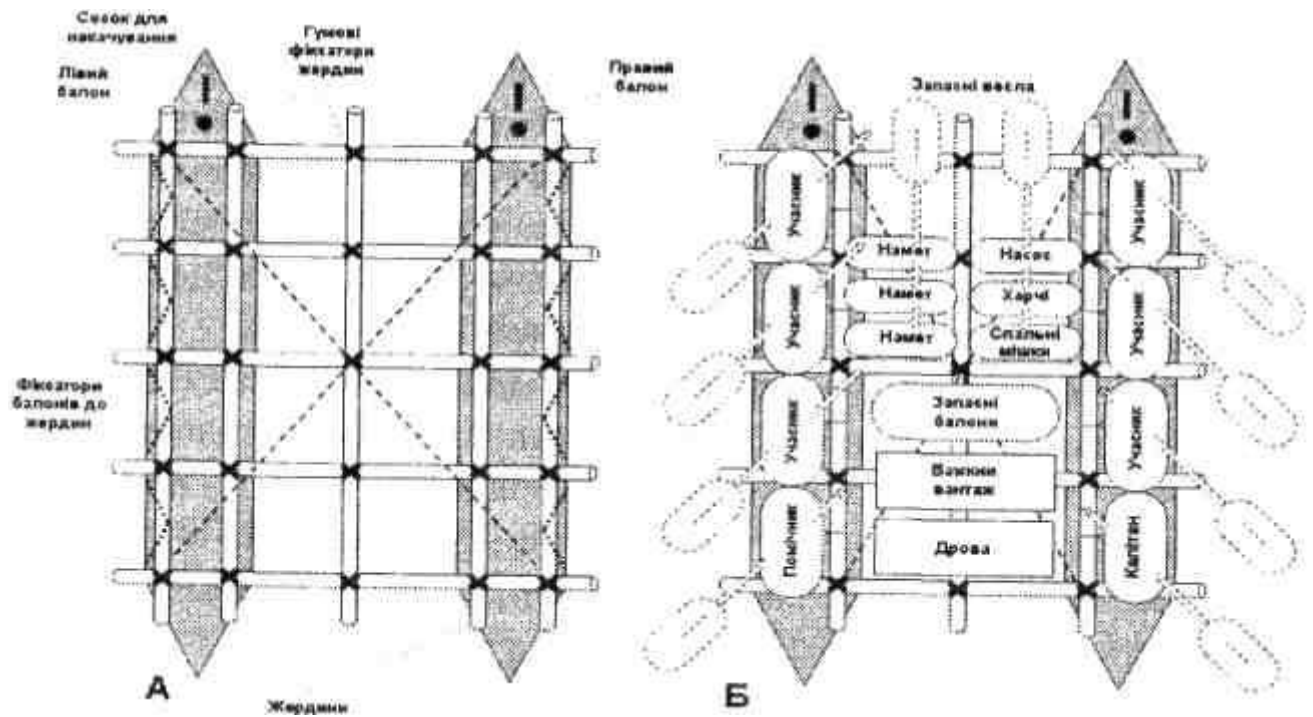
Рис. 6.1. Катамаран а - будова катамарану, б - схема розміщення учасників подорожі та вантажів
