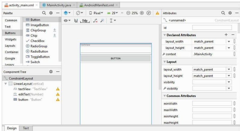
Рис. 1.10 – Інтерфейс програми
