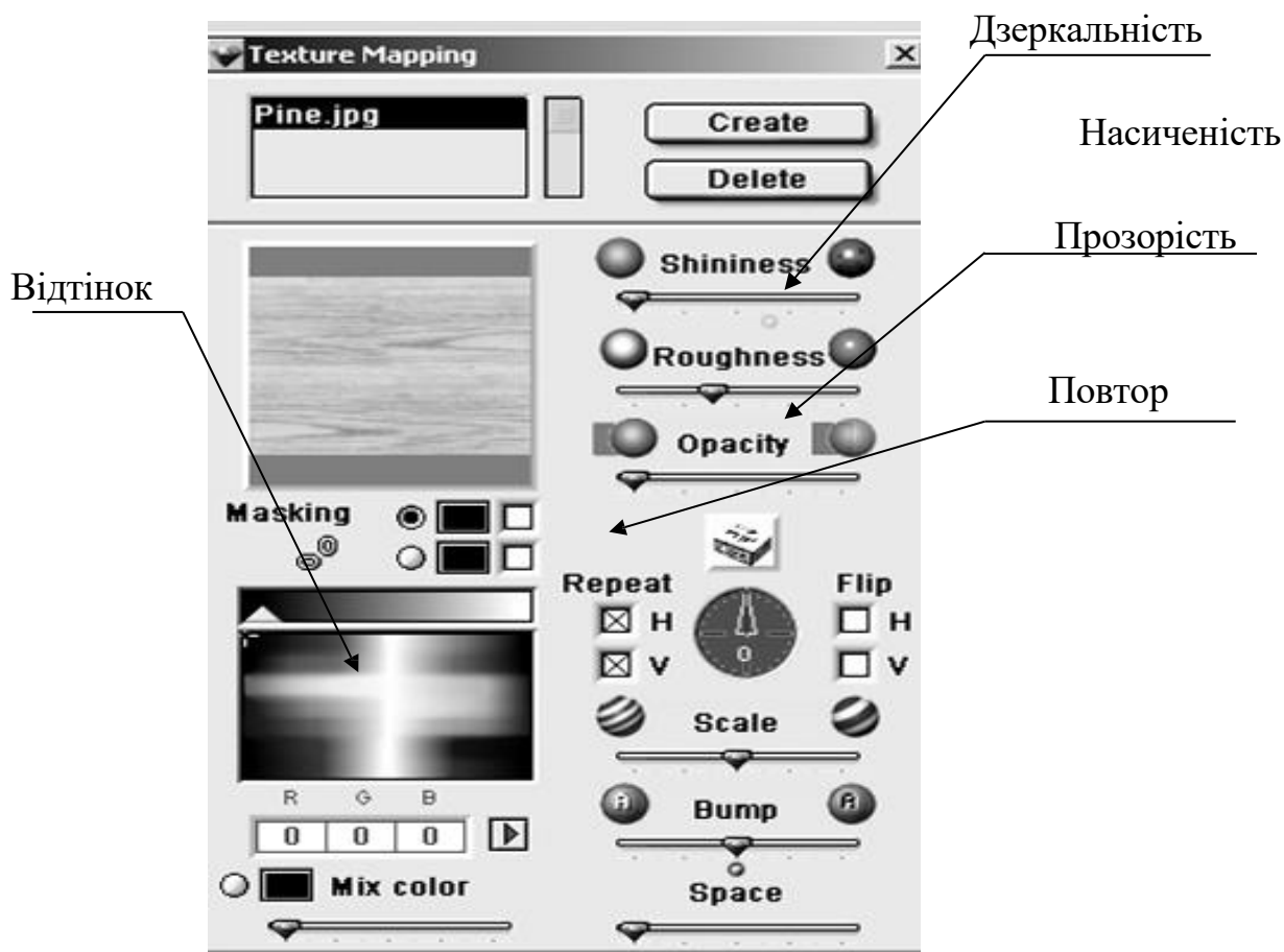
Малюнку 4.12.6– Вікно установки ефектів покриття
