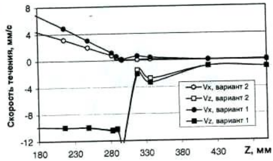
Рисунок 5.8 – Зміна швидкості металу уздовж осі пресування, одержана за допомогою тривимірної моделі
