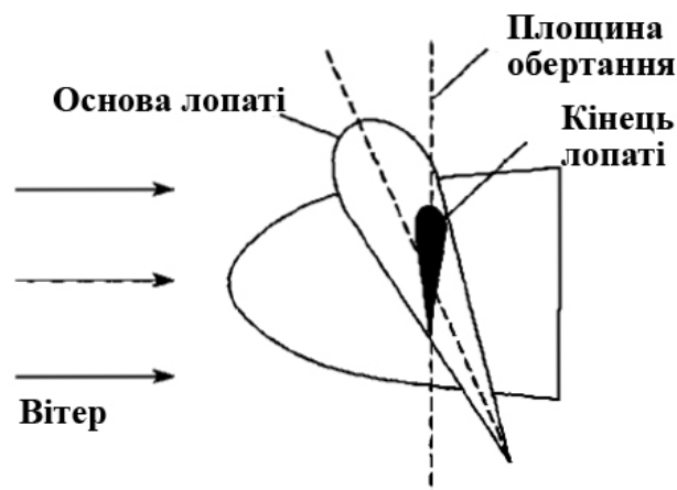
Рис. 8.10. Зовнішній вид профілю крила зі stall-регулюванням
