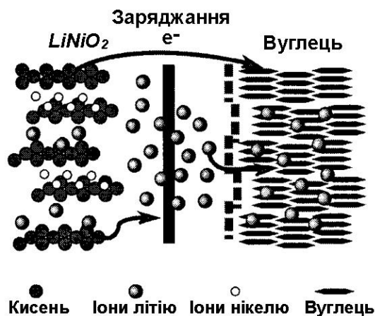
Рис. 2.5. Процес зарядження Li-іон акумулятора
