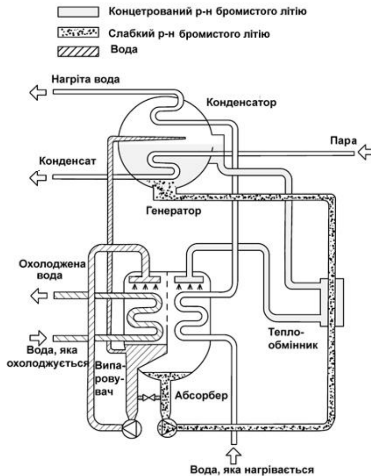
Рис. 5.4. АТН з паровим обігрівом генератора
