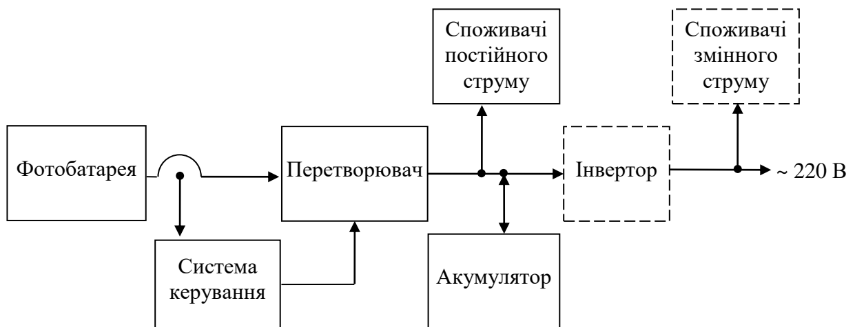
Рис. 7.8. Автономне джерело живлення на основі фотобатарей
