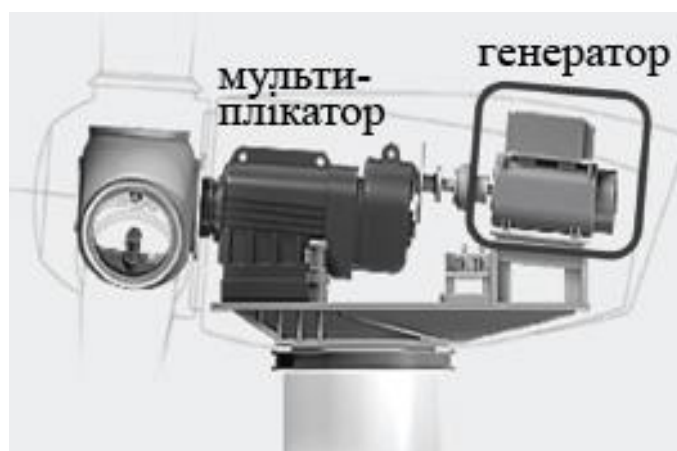
Рис. 8.8. Схema з'єднання валу вітроколеса, мультиплікатора і генератора
