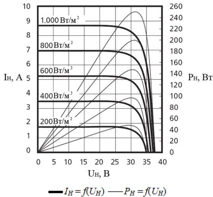
Рис. 7.7. Сімейство ВАХ і кривих потужності фотобатарей
