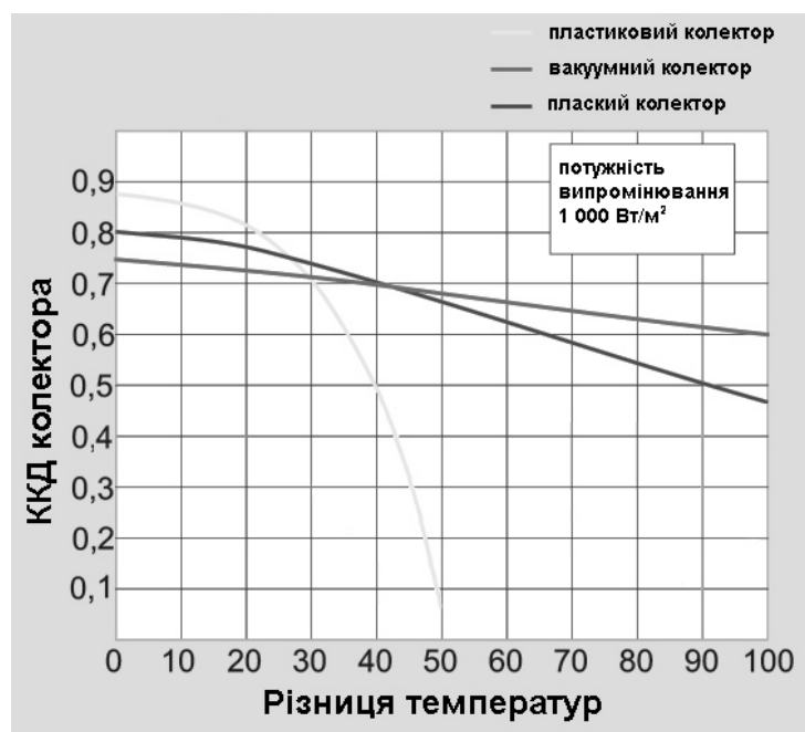
Рис. 6.9. Типова залежність ККД сонячних колекторів
