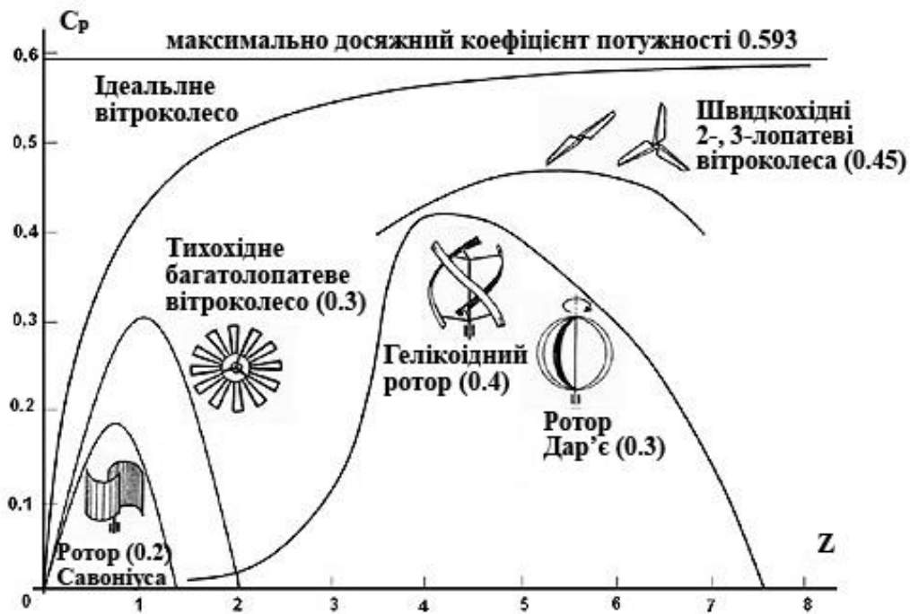
Рис. 8.11. Значення коефіцієнту потужності різних типів вітроколес
