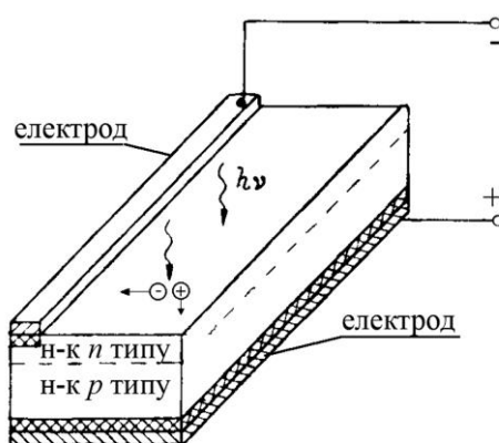
Рис. 7.4. Напівпровідниковий фотоелемент
