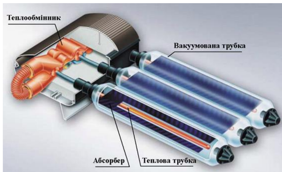
Рис. 6.8. Вакуумний колектор з тепловою трубкою
