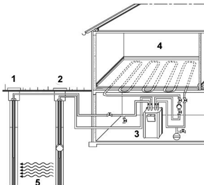
Рис. 5.2. Конструкція системи опалення на основі ПТН типу вода-вода
