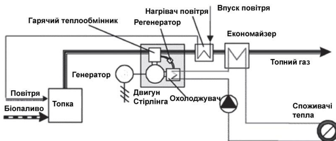
Рис. 4.10. Схема установки з двигуном Стірлінга
