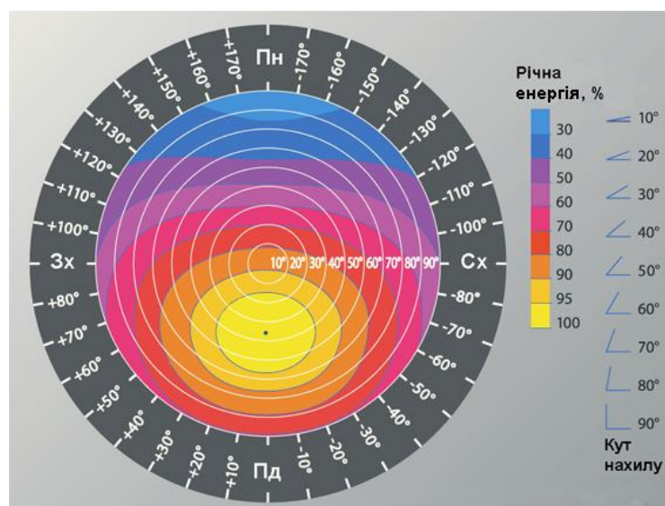
Рис. 6.4. Вплив орієнтації геліоустановки на кількість отриманої енергії
