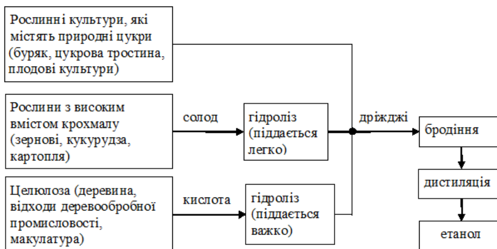
Рис. 3.2. Узагальнена схема отримання етанолу
