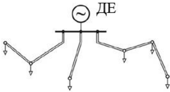
Рис. 9.3. Мережа з резервуванням лінії електропередач
