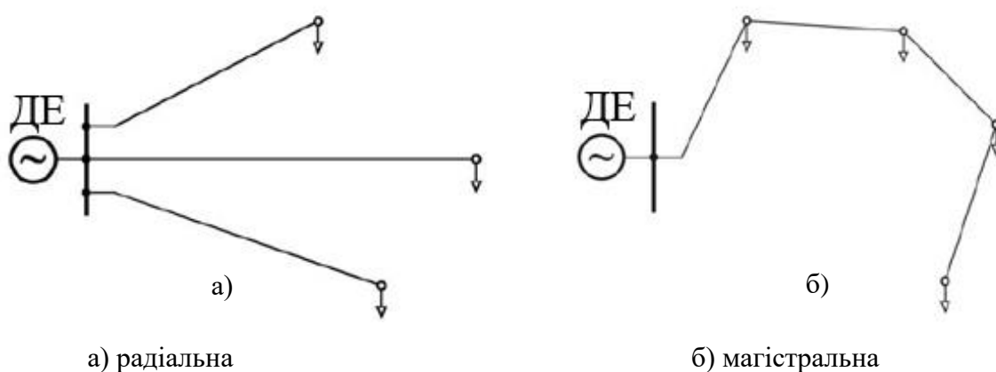
Рис. 9.2. Розімкнена конфігурація мережі
