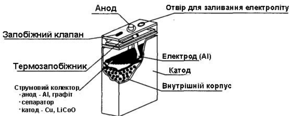
Рис. 2.6. Корпус Li-іон акумулятора
