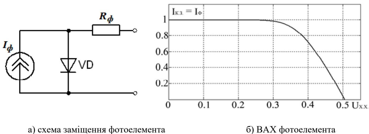
Рис. 7.5. Характеристики фотоелемента
