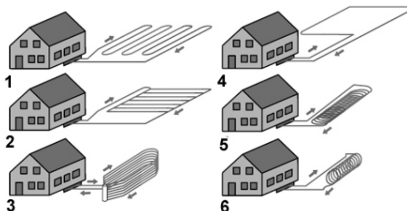
Рис. 5.3. Типи ґрунтових колекторів
