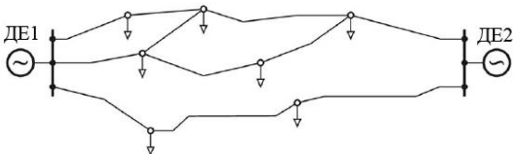
Рис. 9.6. Багатоконтурна конфігурація електромережі
