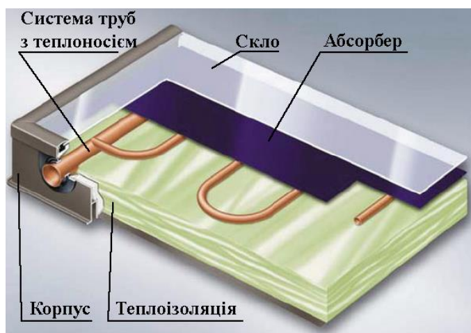
Рис. 6.6. Конструкція плоского колектора
