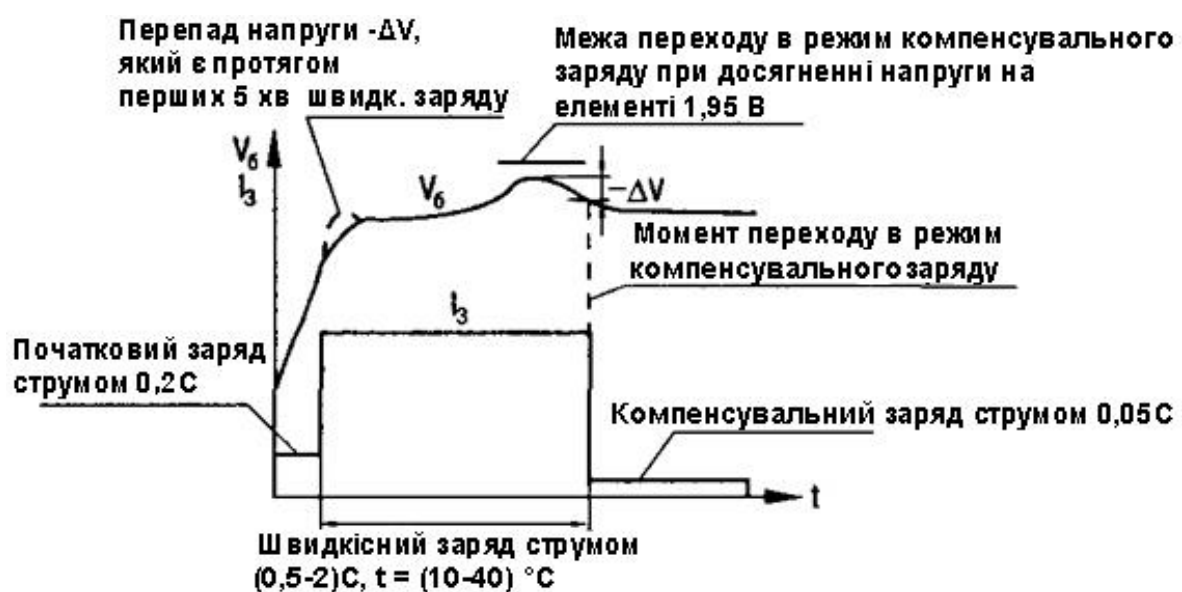
Рис. 2.4. Метод від'ємного \Delta V -заряду
