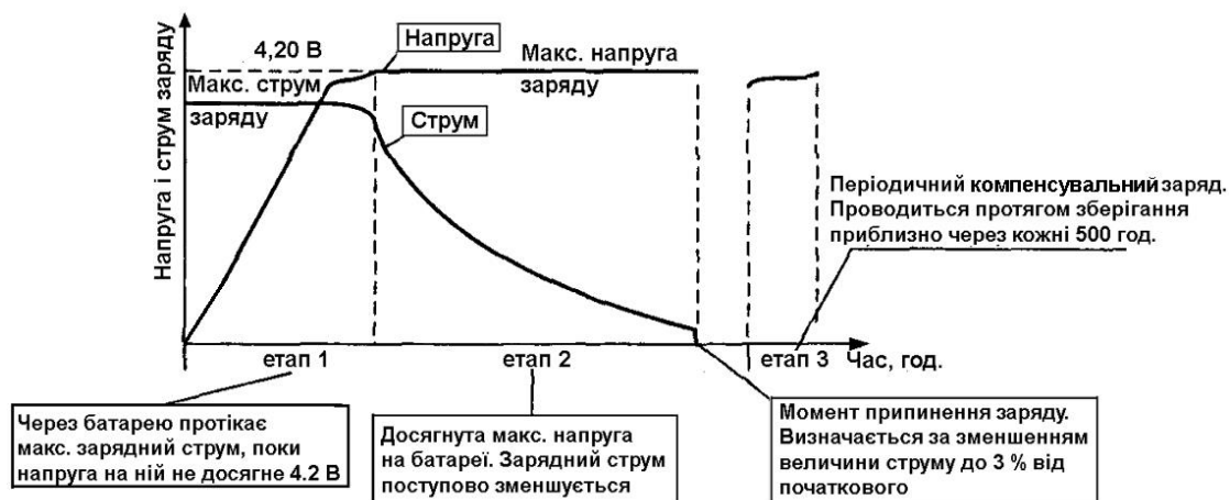
Рис. 2.7. Діаграма заряджання Li-іон акумулятора
