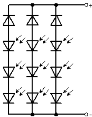
Рис. 7.6. Фотобатарея
