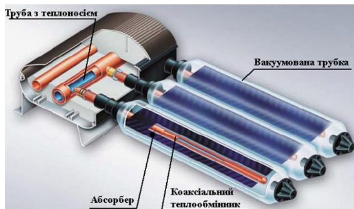
Рис. 6.7. Конструкція вакуумного колектора
