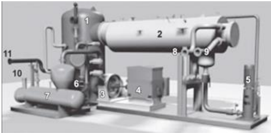
Рис. 4.7. Когенератор на основі ОЦР
