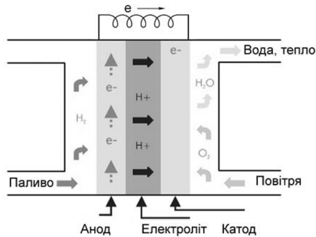
Рис. 4.11. Паливний елемент з протонообмінною мембраною
