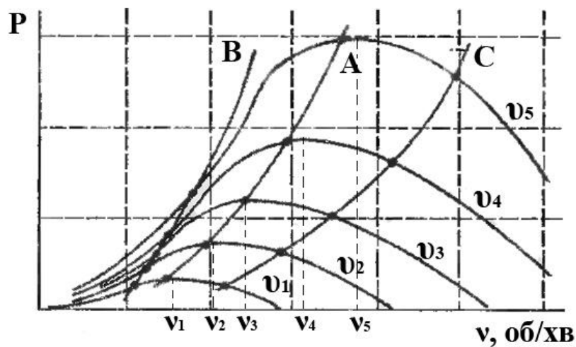
Рис. 8.12. Суміщені характеристики потужності вітродвигуна і генератора
