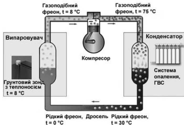
Рис. 5.1. Конструкція ПТН
