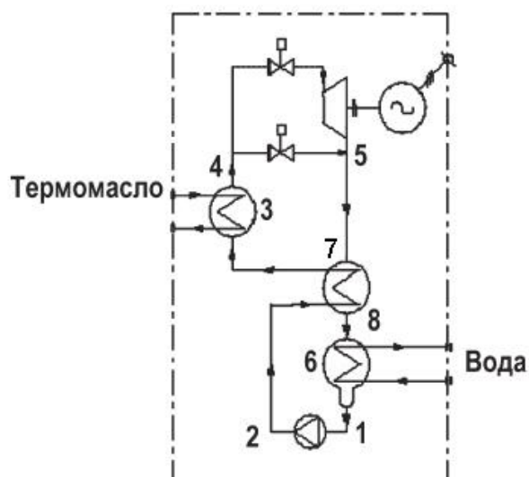
Рис. 4.8. Технологічний цикл установок з ОЦР
