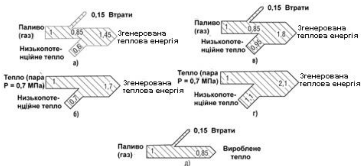
а) АТН на газоподібному паливі, б) АТН на водяній парі, в) двоступеневий АТН на газоподібному паливі, г) двоступеневий АТН на водяній парі, д) газова котельня Рис. 5.5. Порівняльна характеристика втрат у АТН і газовій котельні
