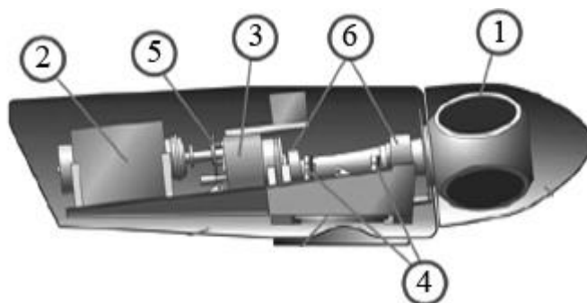
Рис. 8.7. Взаємне розміщення агрегатів у гондолі
