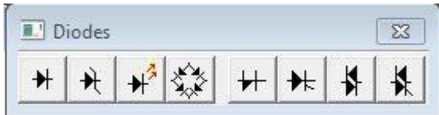
Рисунок 4 – Вкладка Diodes
