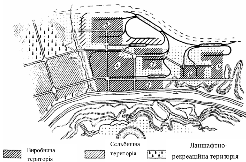
Рис. 5.6 - Схема розміщення промислових підприємств різних класів шкідливості: 1- підприємства I класу, підприємства II класу, підприємства III класу, підприємства IV та V класів.
