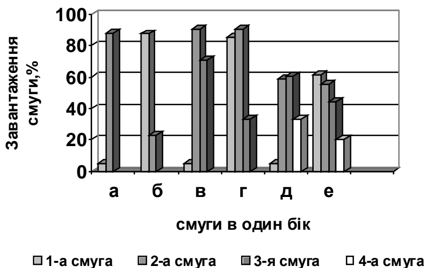
Рис. 11.2 - Діаграма завантаження проїзної частини в «годину пік» у випадку, коли на крайній правій смузі:
