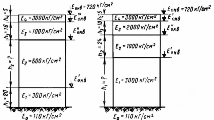
Рис. 13.4 - Розрахункові схеми
