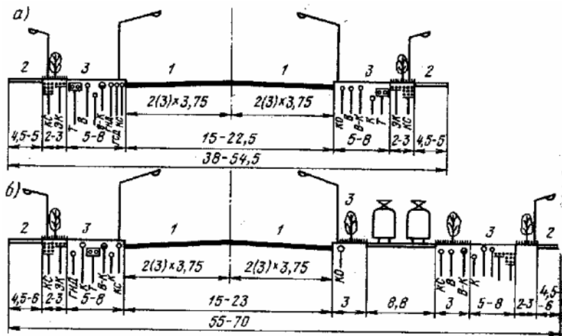
Рис. 12.3 - Поперечні профілі районної магістральної вулиці: а - без трамвайного полотна; б - з відокремленими трамвайним полотном; 1—основна проїзна частина; 2—тротуари; 3—смуги зелених насаджень
