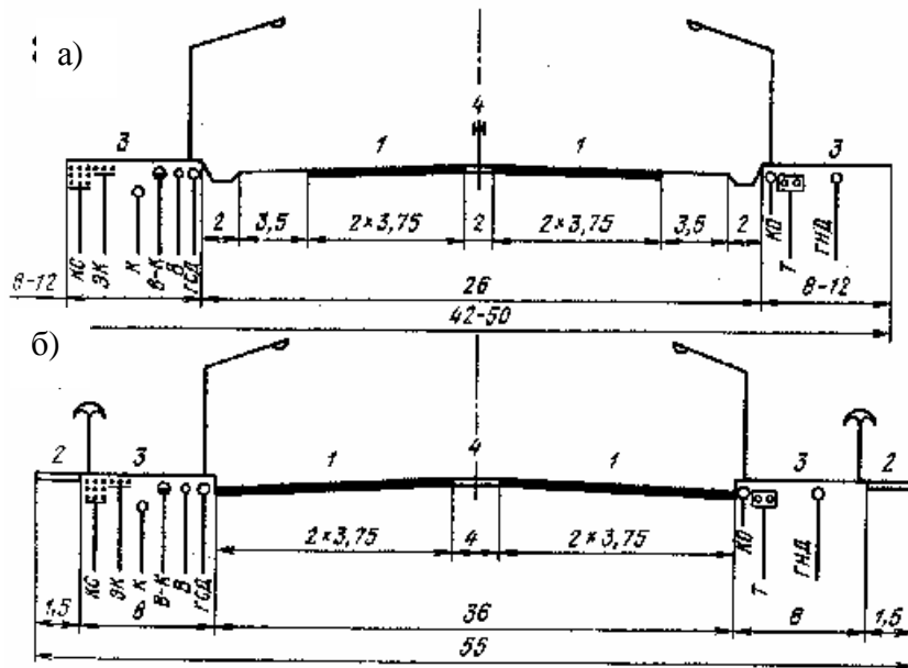
Рис. 12.4 - Поперечні профілі доріг вантажного руху; а – поза забудовою; б – у зоні забудови; 1 – проїзна частина; 2 – тротуари; 3 – смуги зелених насаджень; 4 – центральна розподільна смуга
