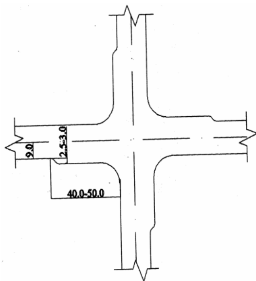
Рис. 10.2 - Приклади деяких схем руху на перехрестях
