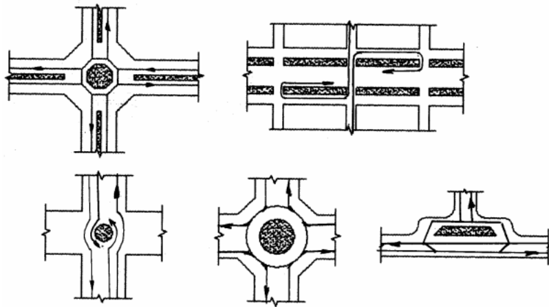
Рис. 10.2 - Приклади деяких схем руху на перехрестях
