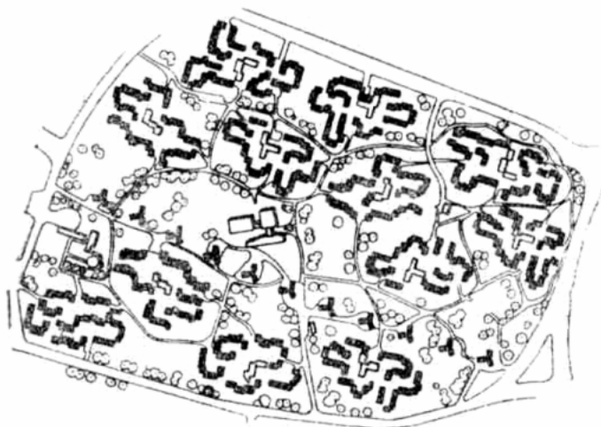
Рис. 4.5- Вільне розташування житлових груп серед зелених насаджень. Проект забудови району Венузю в м. Матера (Італія).
