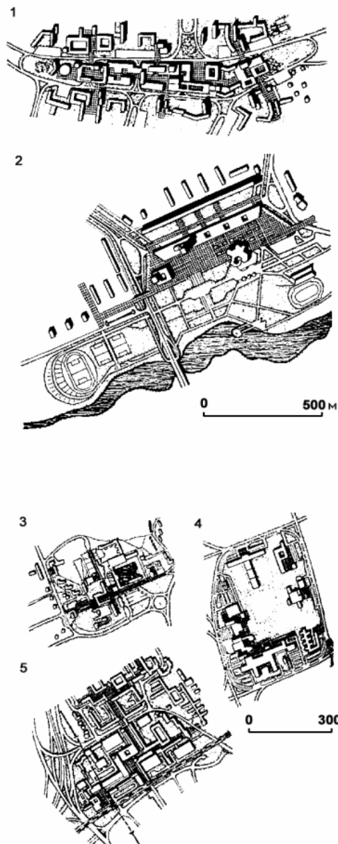
Рис. 7.4 - Форми плану загальних центрів - лінійна: 1 – Кан-Ерувіль, 2 – Зеленоград; компактна: 3 – Хельсінкі - Тапіола, 4 –Кельн - Харвейлер, 5 –Траси, Квебек.
