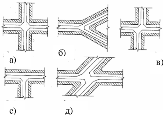
Рис. 10.1 - Типи перехрещень:
