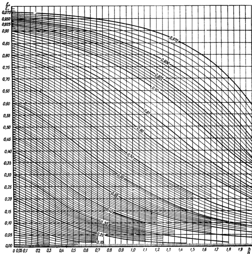
Рис. 13.3 - Номограма для розрахунку дорожнього одягу
