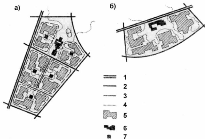
Рис. 4.3 - Схема дорожньої мережі житлових районів: а – житловий район, що членується на мікрорайони; б – житловий район у вигляді збільшеного мікрорайону; 1 – міська швидкісна автодорога, 2 – магістральна вулиця міського призначення, 3 – те ж районного призначення, 4 - житлова вулиця, 5 – мікрорайонні проїзди, 6 – пішохідні доріжки, 7 – територія центру житлового району, 8 – зелені насадження.
