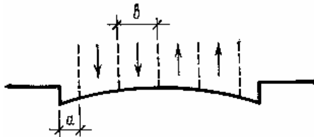
Рис. 12.6 - Розрахунок ширини проїзної частини
