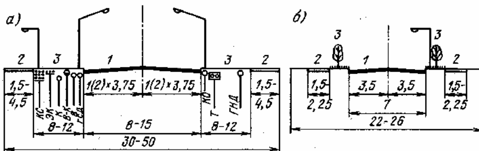
Рис. 12.4 - Поперечні профілі доріг вантажного руху; а – поза забудовою; б – у зоні забудови; 1 – проїзна частина; 2 – тротуари; 3 – смуги зелених насаджень; 4 – центральна розподільна смуга
