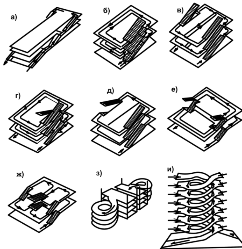
Рис. 10.12 – Найбільш поширені типи рамп. а – прибудовані прямолінійні одно смугові рампи; б – вбудовані прямолінійні двосмугові рампи; в – те ж, одно смугові рампи; г – те ж, рампи, що перехрещуються; д – прямолінійні одно смугові рампи; е – одно смугові напіврампи; ж – те ж, комбіновані; з – прибудовані криволінійні одно смугові рампи; и – односмугова еліптична рампа
