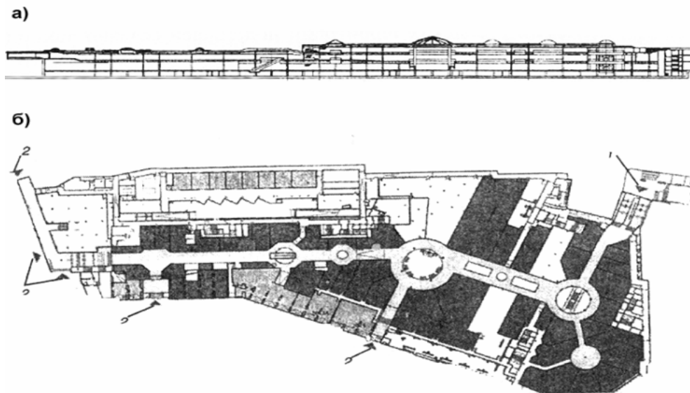
Рис. 2.14 - Підземний торговіельно-рекреаційний комплекс на Манежній площі в Москві: а – переріз; б – план; 1 – вхід до вестибюля станції; 2 – вхід до станції з площі
