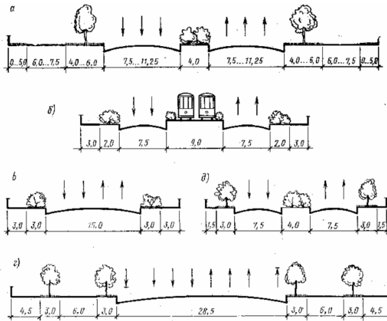
Рис. 12.7 - Поперечні профілі магістральних вулиць
