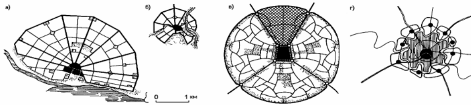
Рис. 2.12 - Первісні форми центричного плану міста: а – план Костроми, б – план Солігаліча (1781 р.), в – теоретична модель англійського нового міста (Л. Кіл, 1961р.), г – концентричний розвиток Парижа.
