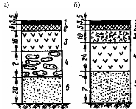
Рис. 13.2 - Приклад схеми конструкції нежорсткого дорожнього одягу
