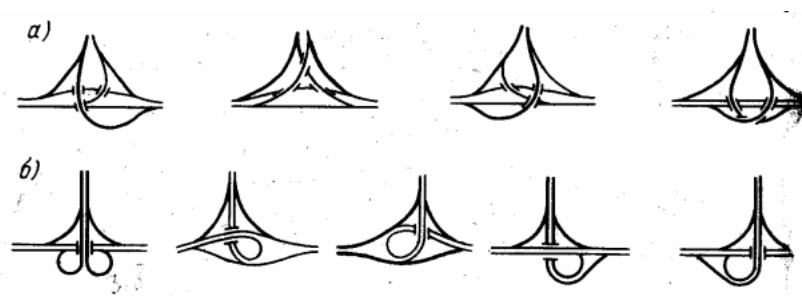
Рис. 10.8 - Повні примикання:
