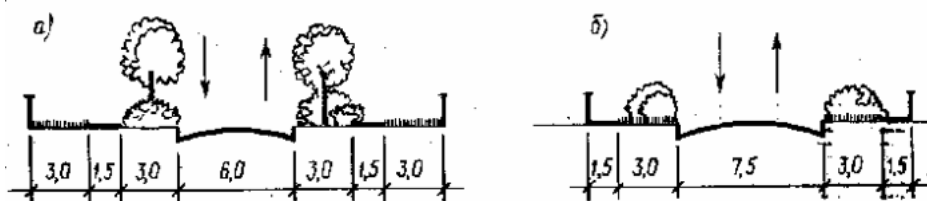
Рис. 12.8 - Поперечні профілі вулиць і доріг місцевого значення
