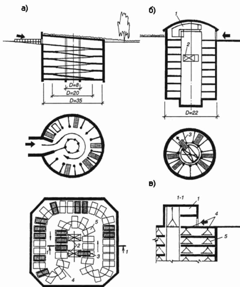
Рис. 4.13 - Підземні гаражі: а – скатно - гвинтового типу; б – те ж роторного з обертовою навколо вертикальної осі кабіною ліфта; в – з підйомником конвеєром-монорейкою; 1 – машинне відділення підйомника; 3 – установлювана машина; 4 – монорейка конвеєра; 5 – платформа для машин.
