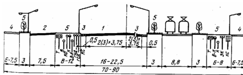
Рис. 12.2 - Поперечний профіль загальноміської магістральної вулиці з відокремленими трамвайними коліями: ЭЖ, Т, КО, КС, К, Т, В – інженерні мережі
