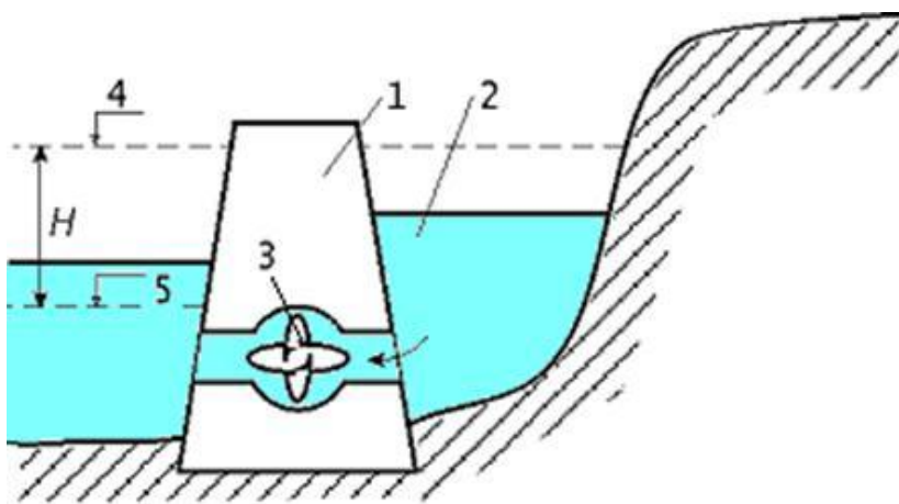
Рис. 5.1 – Принцип роботи приливної електростанції:
