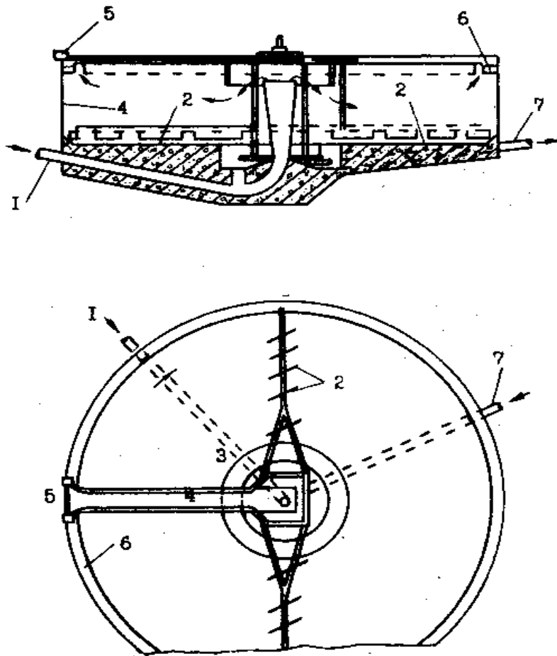
Рисунок 9 – Радіальний відстійник:
