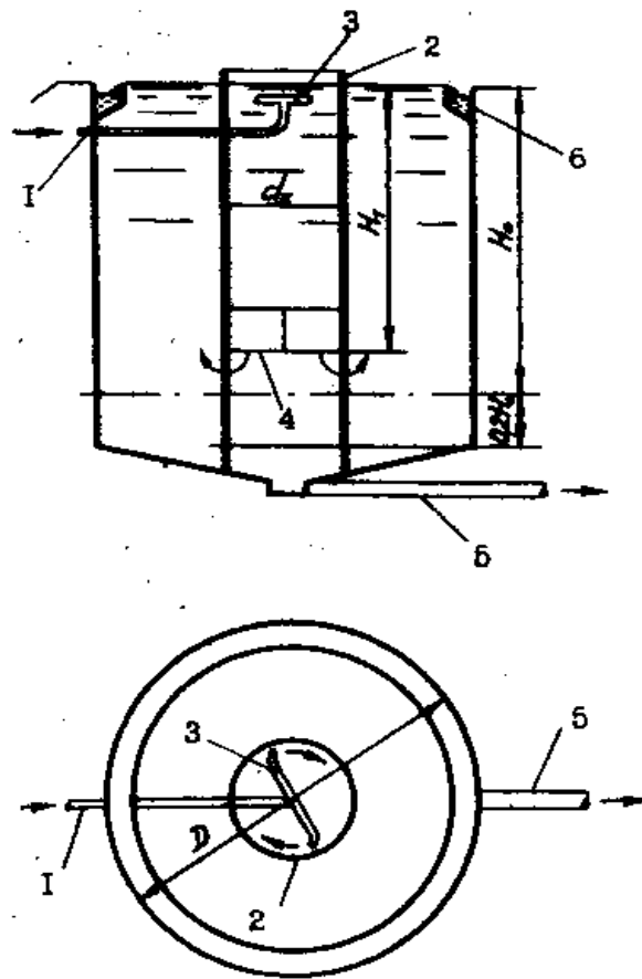
Рисунок 6 - Вертикальний відстійник з водоворотною камерою пластівцеутворення:
