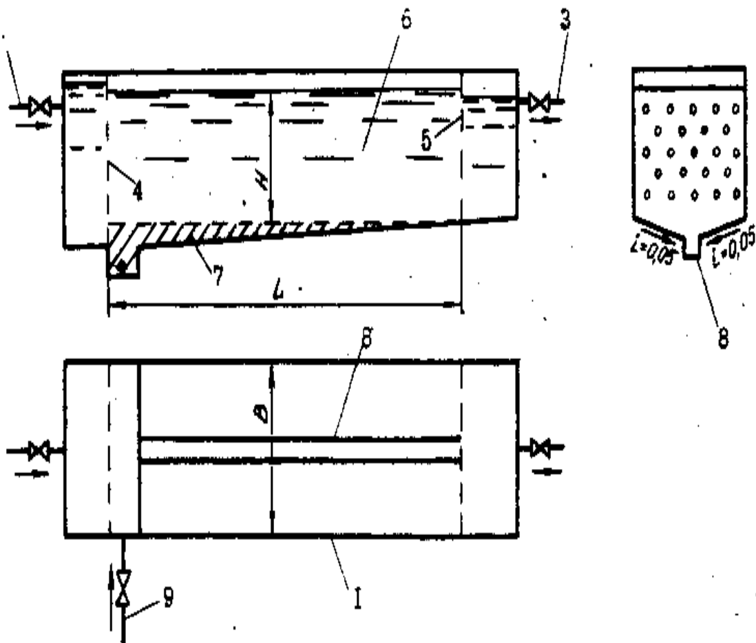
Рисунок 8 – Горизонтальний відстійник:
