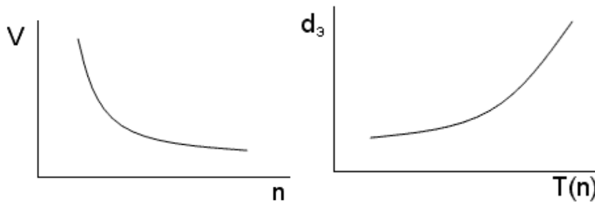
Рисунок 12 – Залежність швидкостей в лотках ( V ) від числа працюючих споруд при Q_p=\text{const} ; залежність крупності пластівців коагулянту ( d_3 ) від часу коагуляції чи від числа працюючих камер пластівцеутворення
