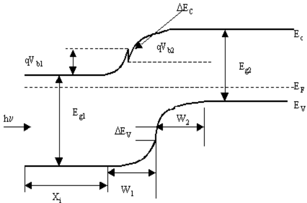
Діаграма енергетических зон n - p-гетеропереходов в стані термодинамічного рівноваги.
